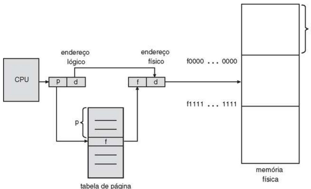
FIGURA 8.7 Hardware de paginação.
