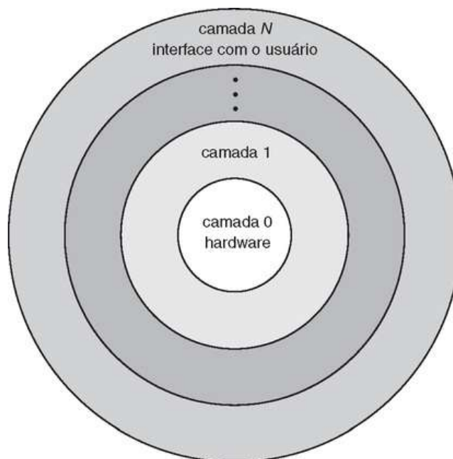
FIGURA 2.14 Um sistema operacional em camadas.
