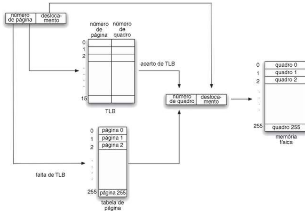
FIGURA 9.34 Representação do processo de tradução de endereços.
