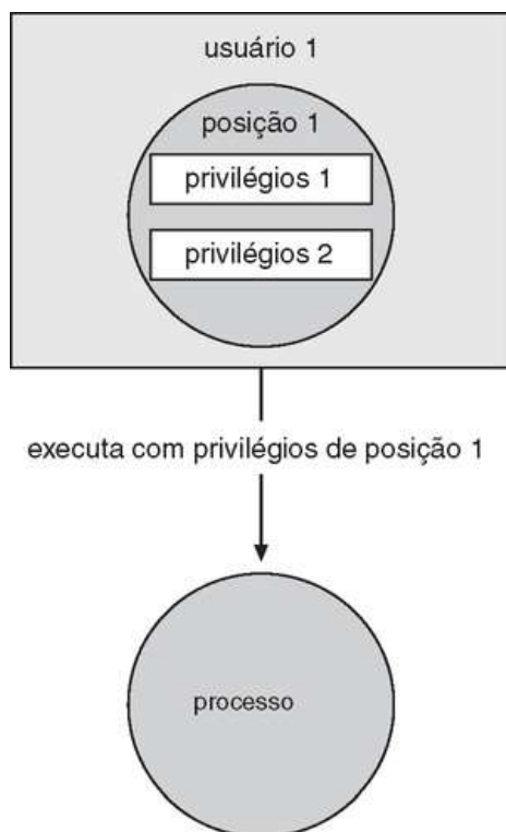
FIGURA 14.8 Controle de acesso baseado em posição no Solaris 10.
