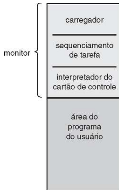
FIGURA 23.2 Layout de memória para um monitor residente.
