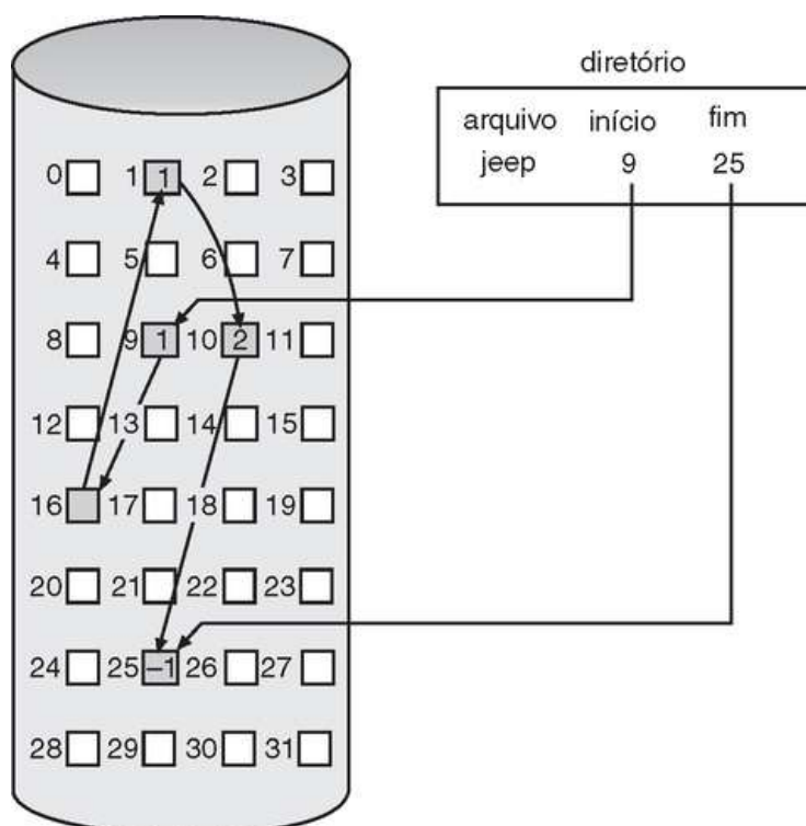
FIGURA 11.6 Alocação interligada do espaço em disco.
