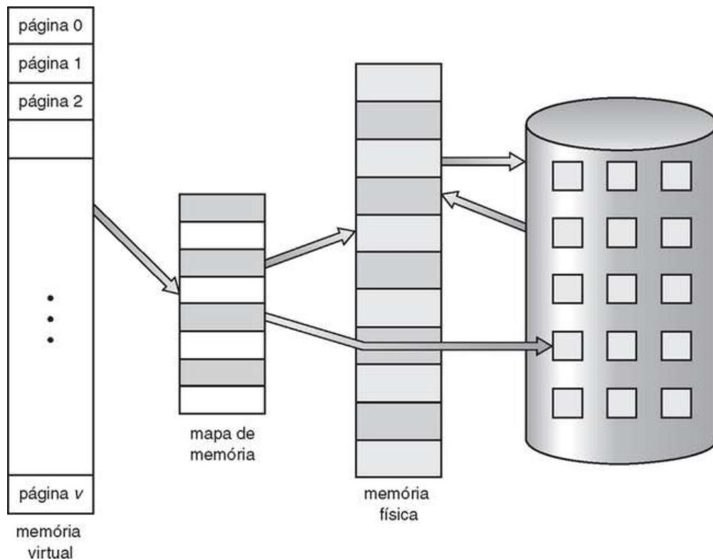
FIGURA 9.1 Diagrama mostrando a memória virtual que é maior do que a memória física.
