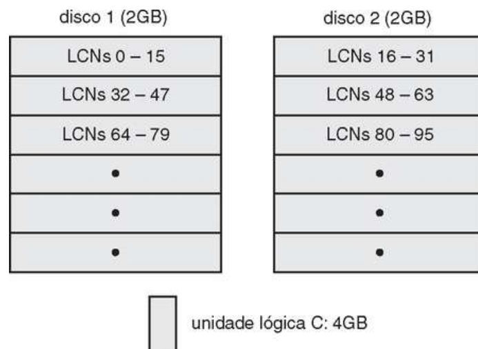
FIGURA 22.8 Stripe set em duas unidades.
