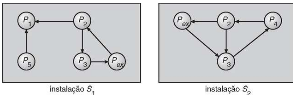
FIGURA 18.6 Grafos de espera locais aumentados da Figura 18.3 .
