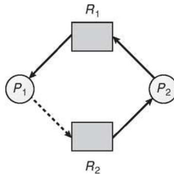
FIGURA 7.10 Um estado inseguro em um grafo de alocação de recursos.
