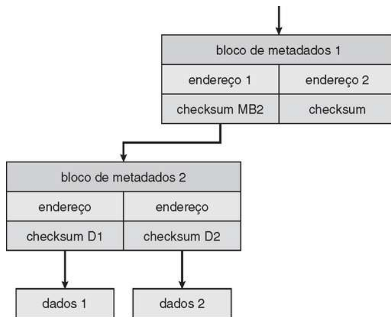
FIGURA 12.13 ZFS verifica a soma de todos os metadados e dados.
