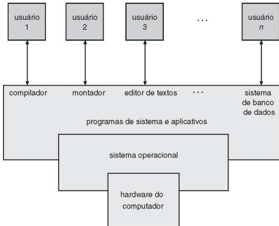
FIGURA 1.1 Visão abstrata dos componentes de um sistema computadorizado.
