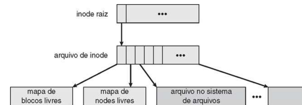
FIGURA 11.16 O layout de arquivo WAFL.
