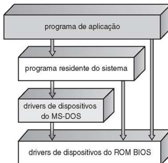
FIGURA 2.12 Estrutura de camadas do MS-DOS.
