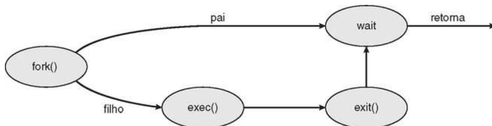
FIGURA 3.11 Criação de processo usando a chamada de sistema fork() .
