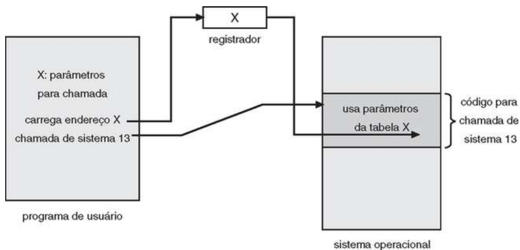
FIGURA 2.7 Passagem de parâmetros como uma tabela.
