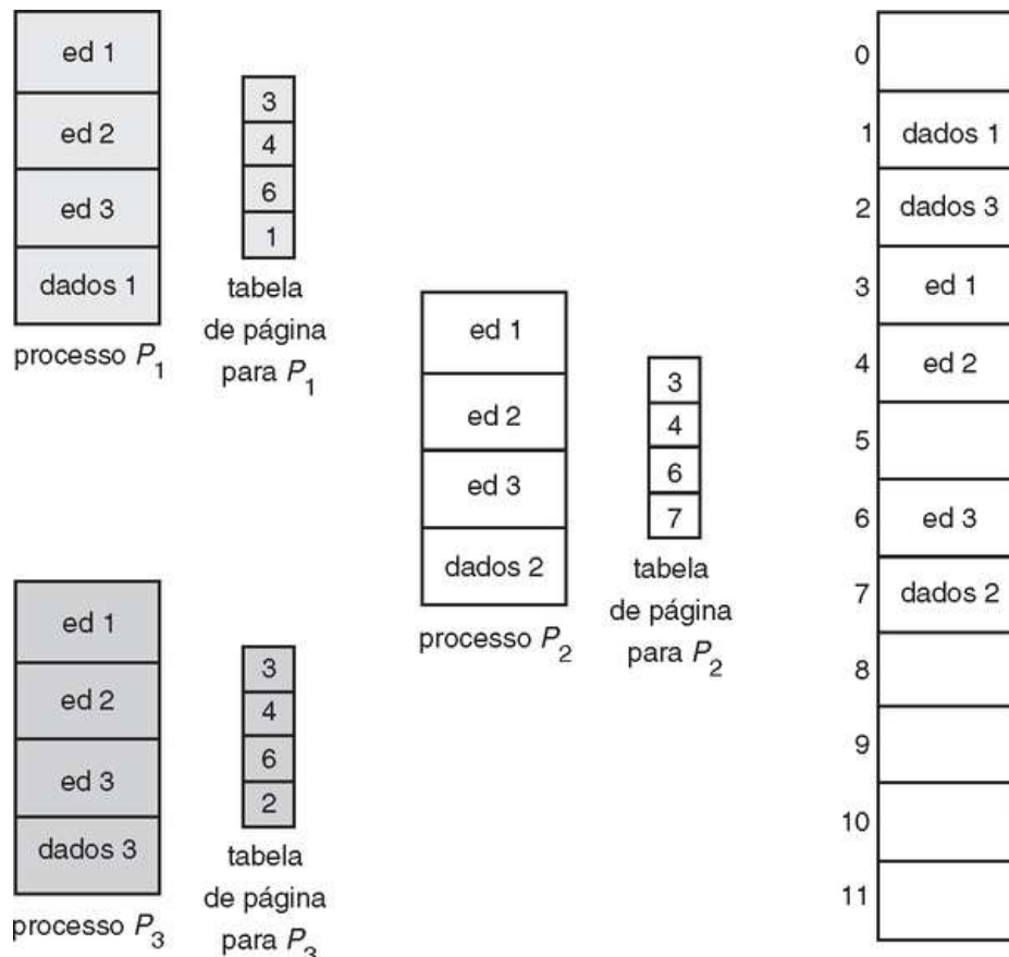
FIGURA 8.13 Compartilhamento de código em um ambiente de paginação.
