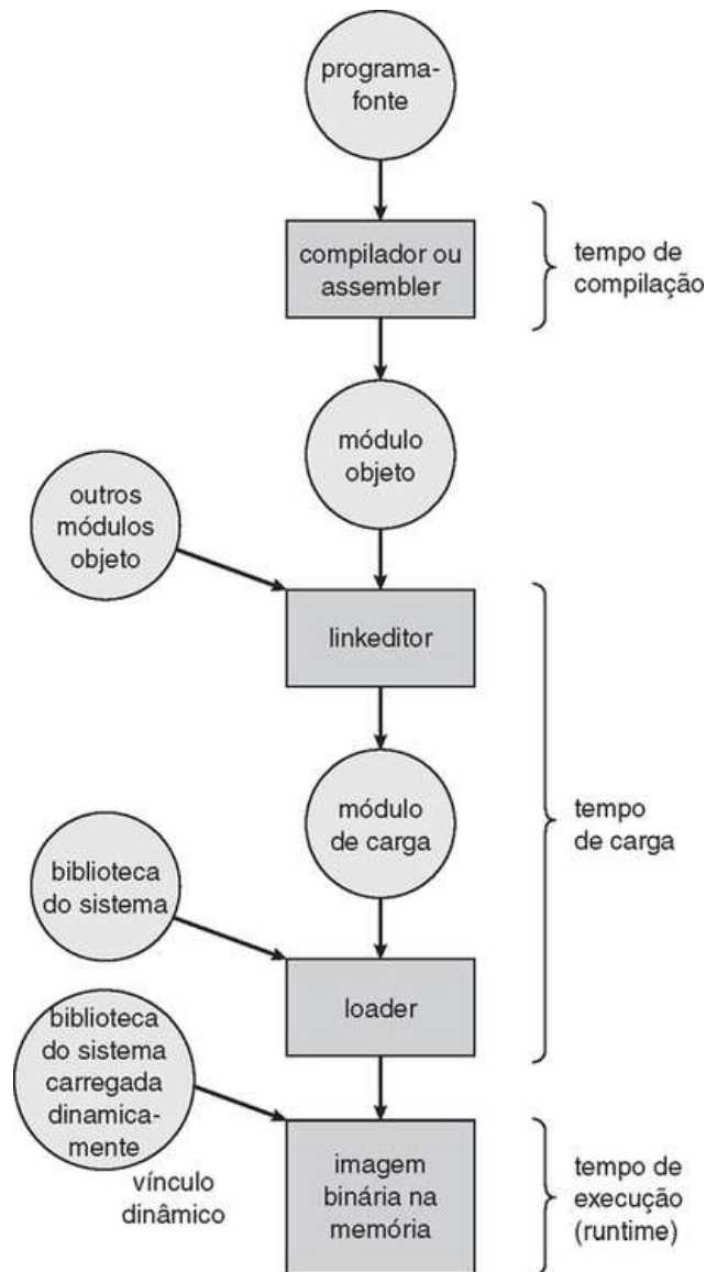
FIGURA 8.3 Processamento de um programa do usuário em múltiplas etapas.
