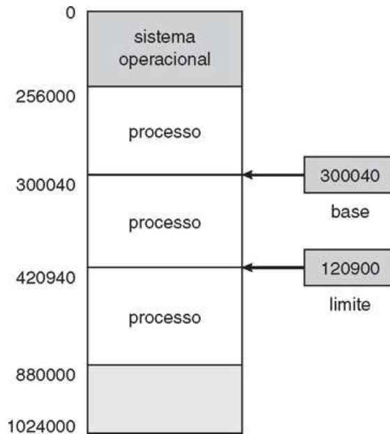
FIGURA 8.1 Um registrador de base e um de limite definem um espaço de endereços lógicos.
