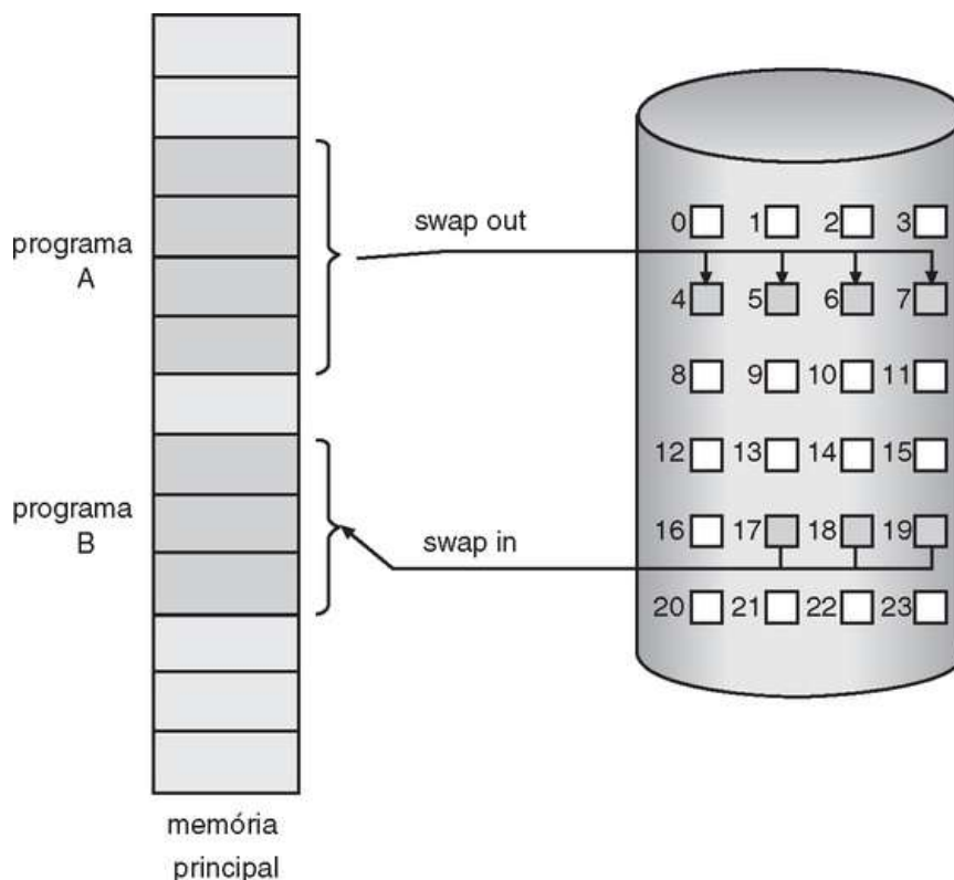
FIGURA 9.4 Transferência de uma memória paginada para o espaço contíguo no disco.
