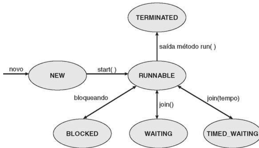
FIGURA 4.12 Estados da thread em Java.
