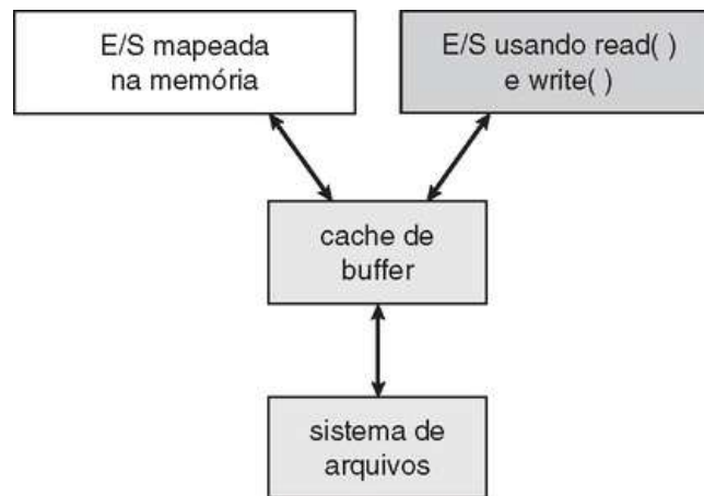
FIGURA 11.12 E/S usando um buffer cache unificado.
