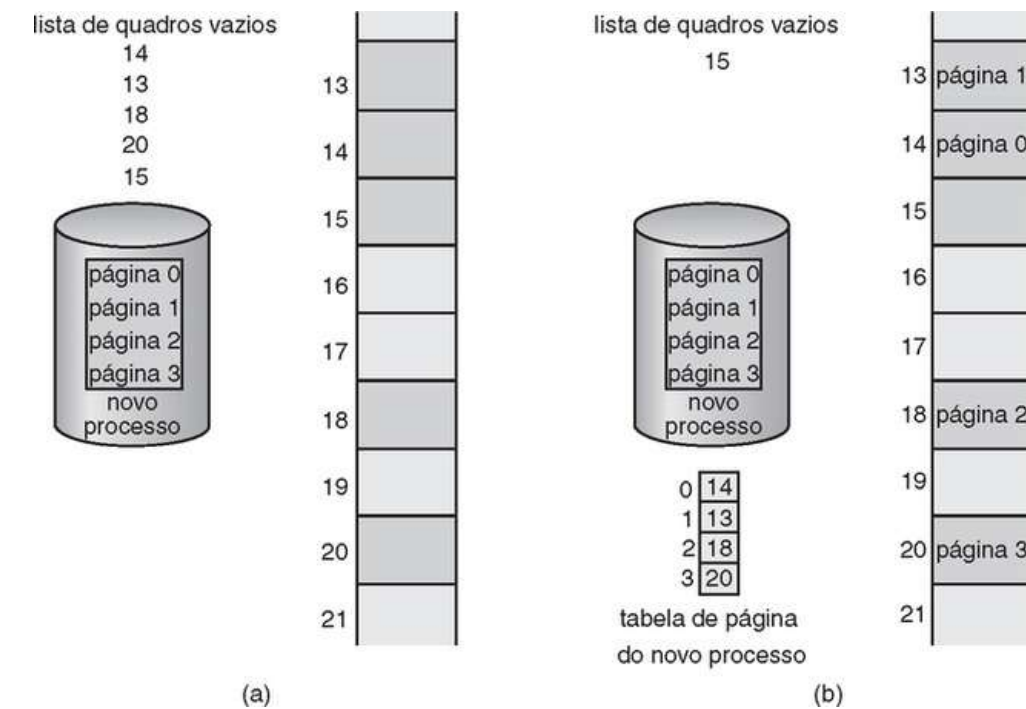
FIGURA 8.10 Quadros vazios. (a) Antes da alocação e (b) após a alocação.
