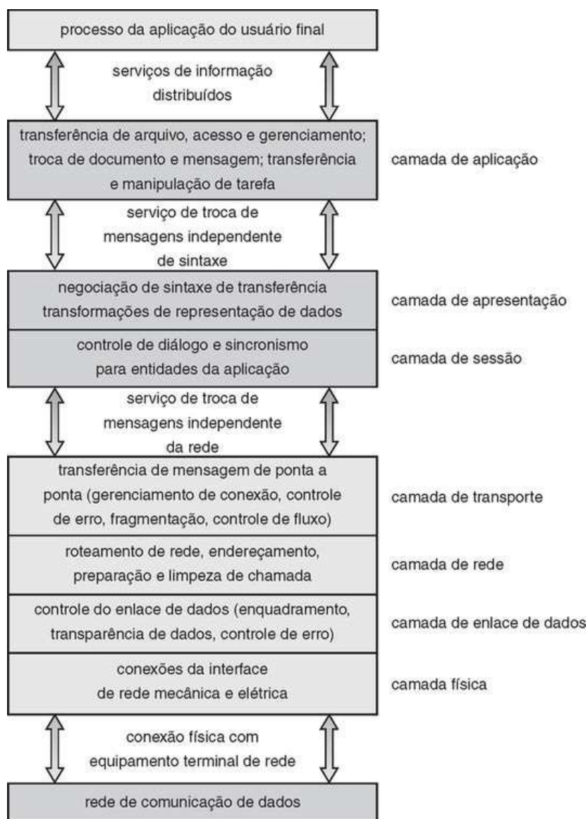
FIGURA 16.7 A pilha de protocolos ISO.
