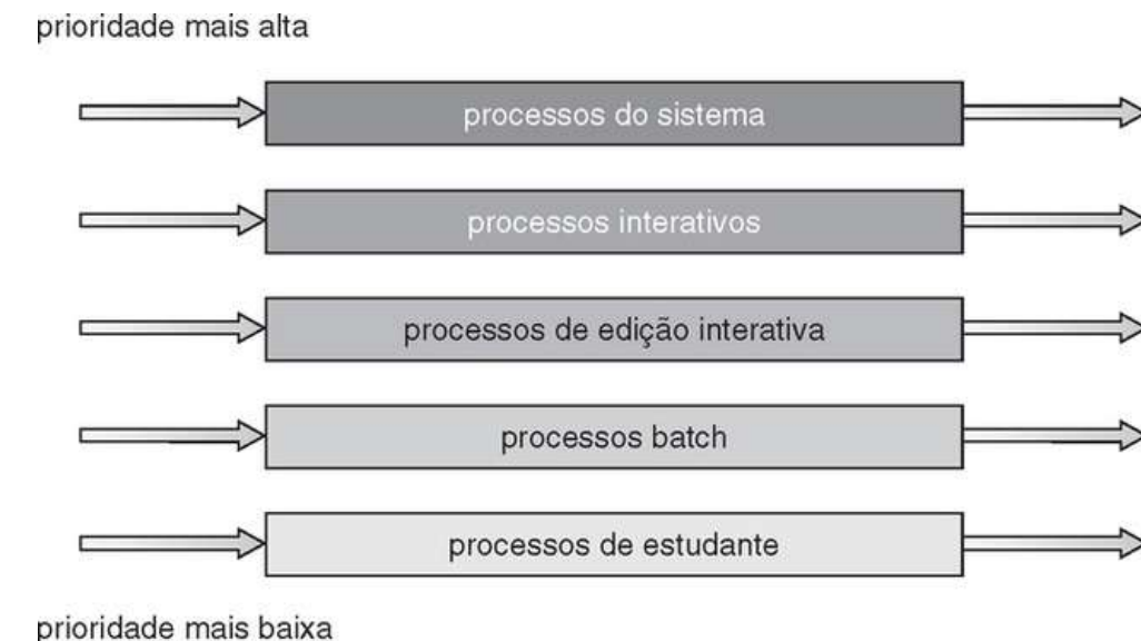
FIGURA 5.6 Escalonamento de multilevel queue.
