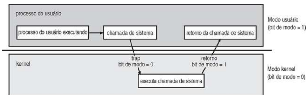
FIGURA 1.10 Transição de modo usuário para modo kernel.
