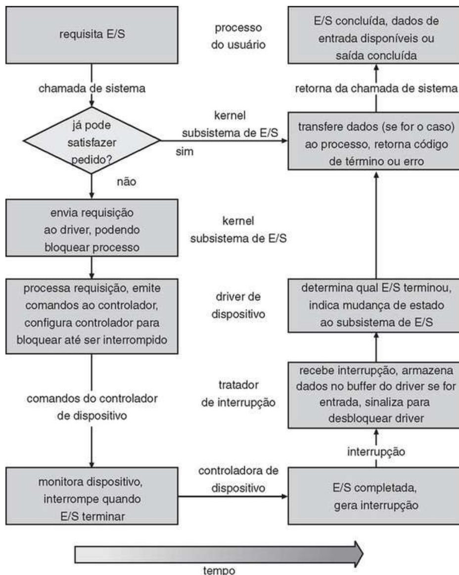
FIGURA 13.13 O ciclo de vida de uma requisição de E/S.
