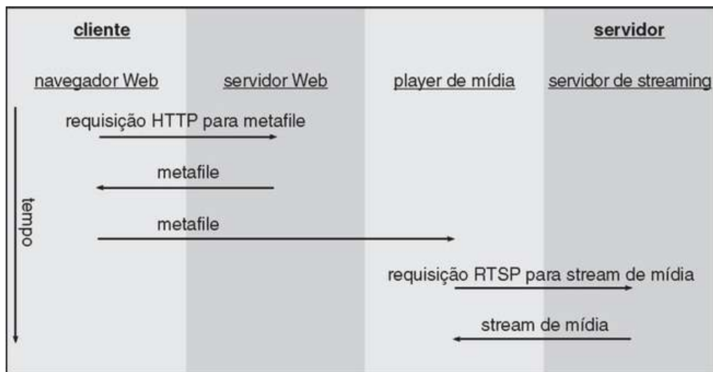
FIGURA 20.3 Protocolo de streaming em tempo real (RTSP).
