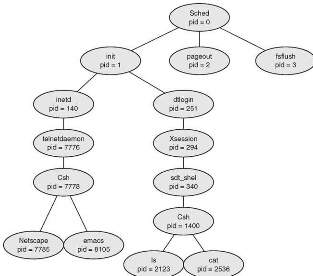
FIGURA 3.9 Uma árvore de processos em um sistema Solaris típico.
