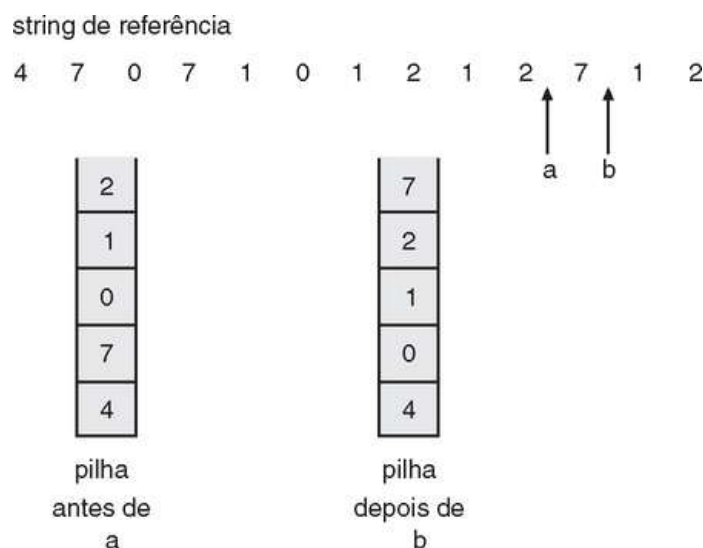
FIGURA 9.16 Uso de uma pilha para registrar as referências de página mais recentes.
