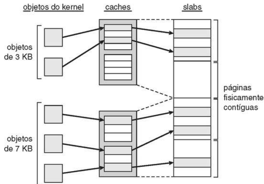
FIGURA 9.27 Alocação de slabs.
