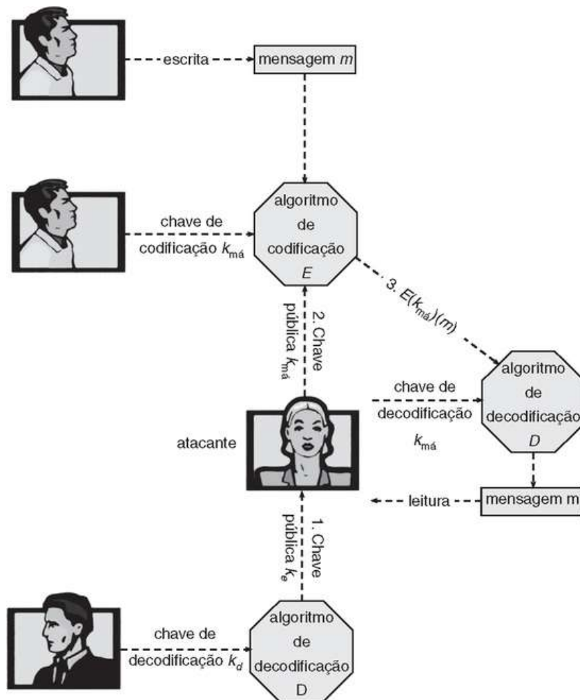
FIGURA 15.9 Ataque de homem no meio na criptografia assimétrica.
