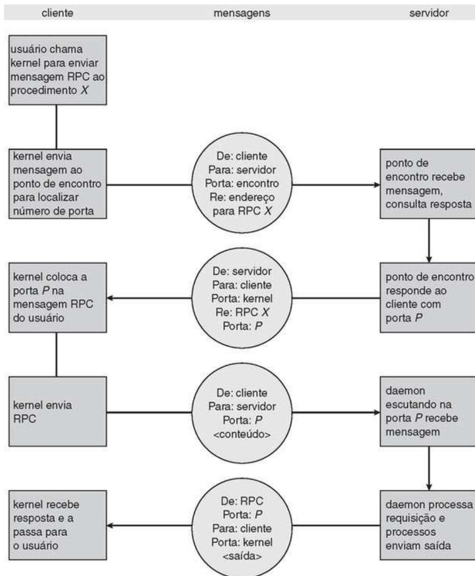
FIGURA 3.28 Execução de uma remote procedure call (RPC).
