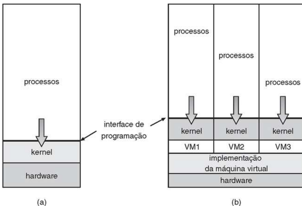
FIGURA 2.17 Modelos de sistema: (a) máquina não virtual e (b) máquina virtual.
