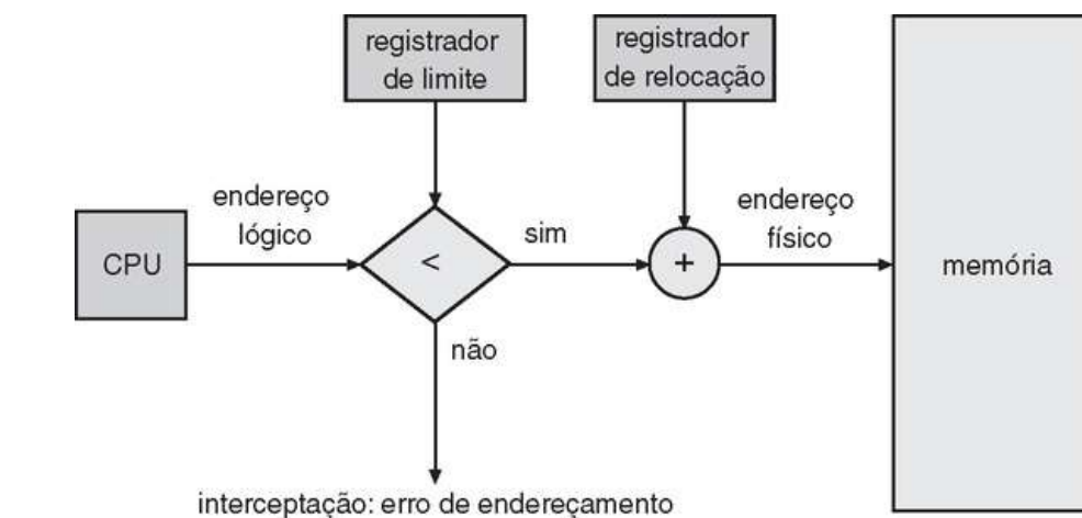
FIGURA 8.6 Suporte do hardware para registradores de relocação e limite.
