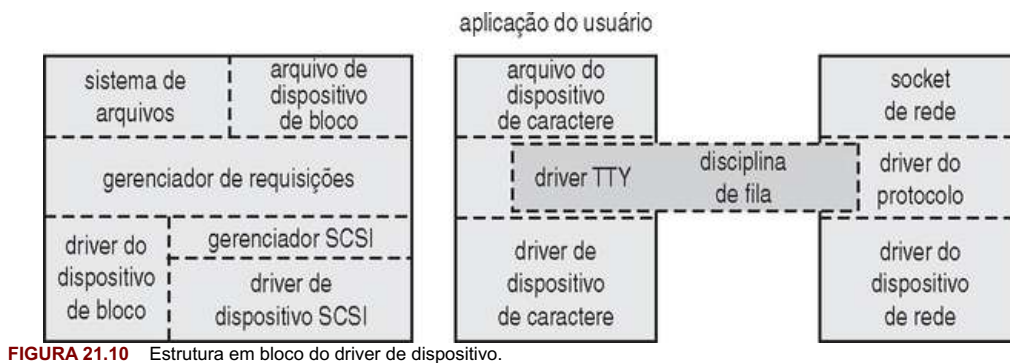
FIGURA 21.10 Estrutura em bloco do driver de dispositivo.
