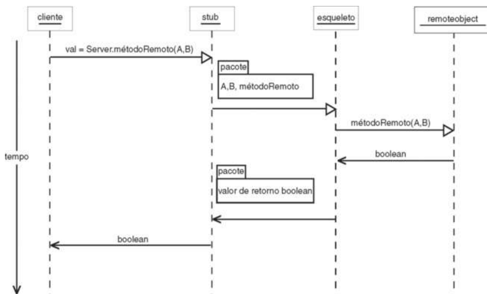
FIGURA 3.30 Parâmetros de empacotamento.
