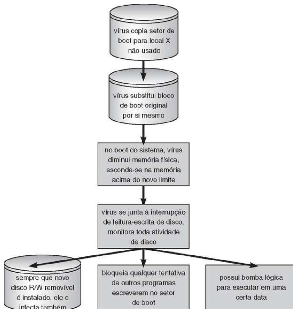
FIGURA 15.5 Um vírus de computador do setor de boot.
