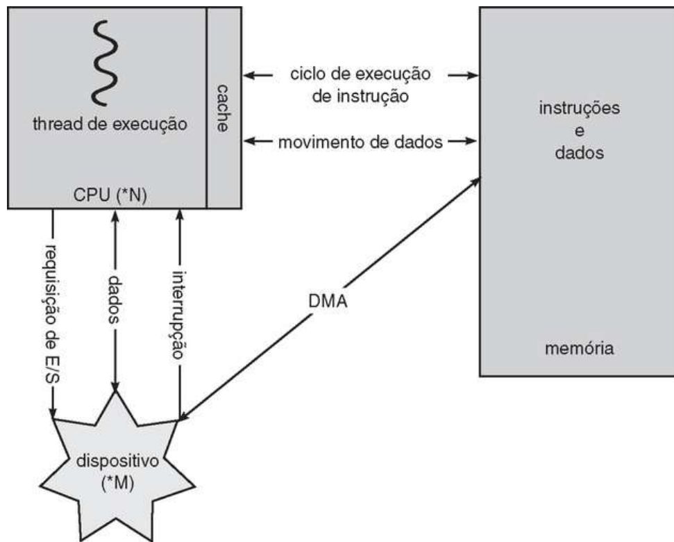
FIGURA 1.5 Como funciona um sistema computadorizado moderno.
