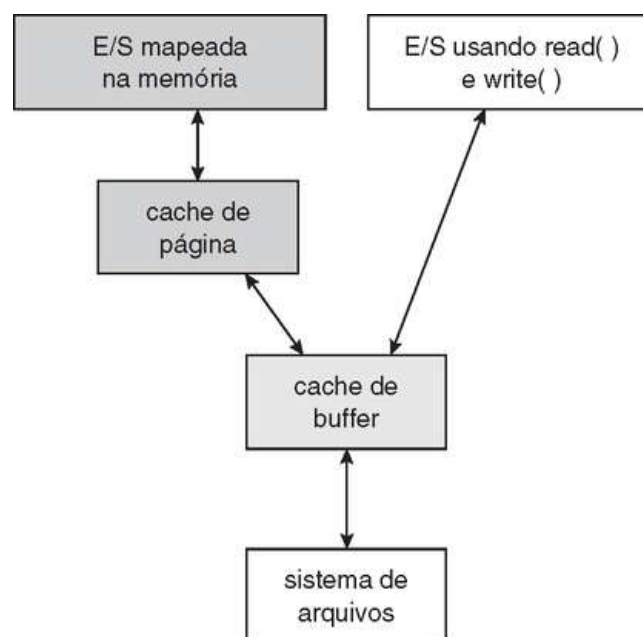
FIGURA 11.11 E/S sem um buffer cache unificado.
