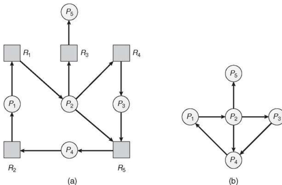
FIGURA 7.11 (a) Grafo de alocação de recursos e (b) grafo wait-for correspondente.
