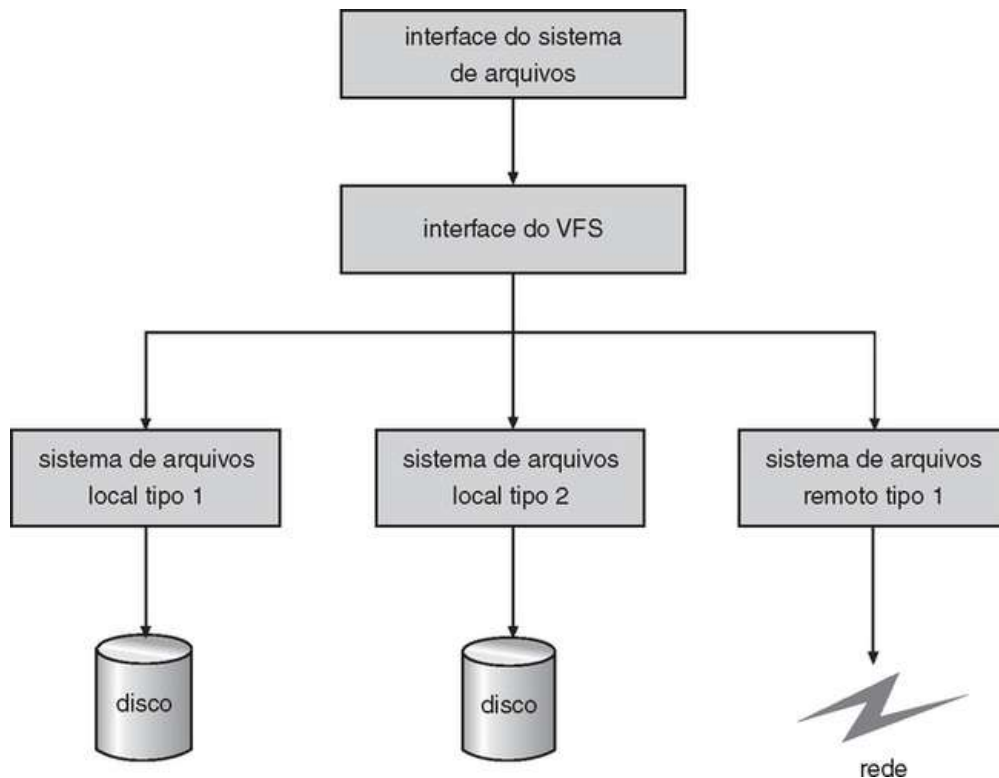
FIGURA 11.4 Visão esquemática do sistema de arquivos virtual.
