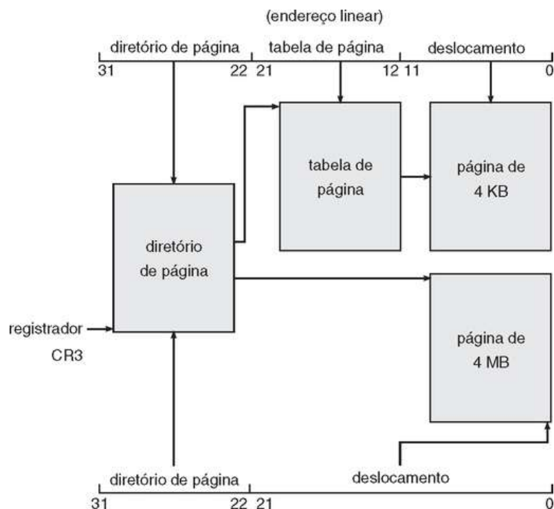
FIGURA 8.23 Paginação na arquitetura Pentium.
