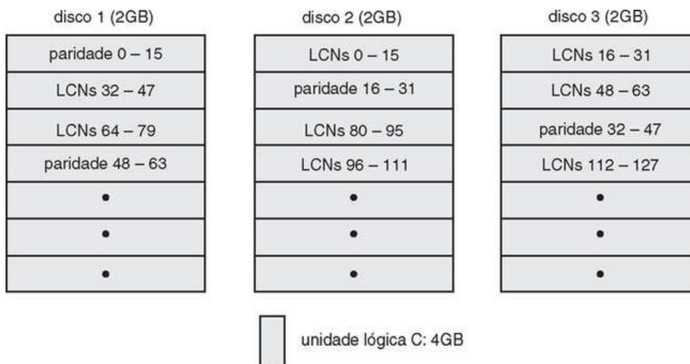
FIGURA 22.9 Stripe set com paridade em três unidades.
