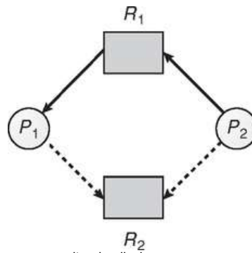
FIGURA 7.9 Grafo de alocação de recursos para evitar deadlock.
