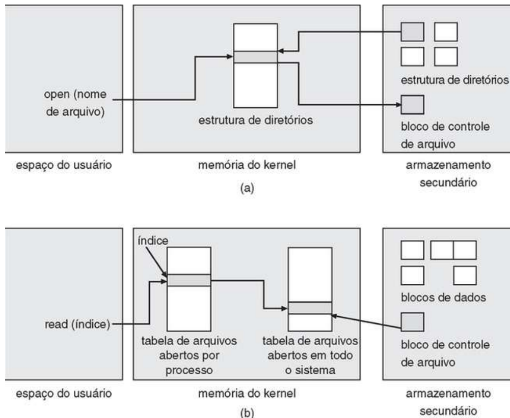
FIGURA 11.3 Estruturas do sistema de arquivos na memória. (a) Abertura de arquivo e (b) leitura de arquivo.
