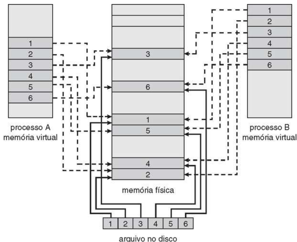
FIGURA 9.23 Arquivos mapeados na memória.
