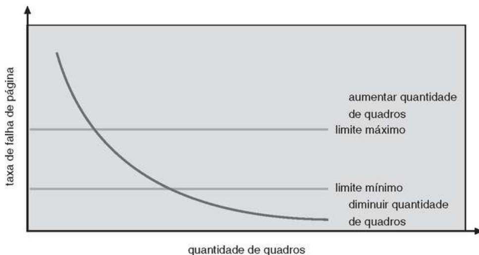
FIGURA 9.21 Frequência de falha de página.
