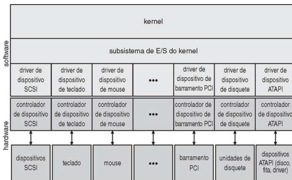
FIGURA 13.6 Uma estrutura de E/S do kernel.
