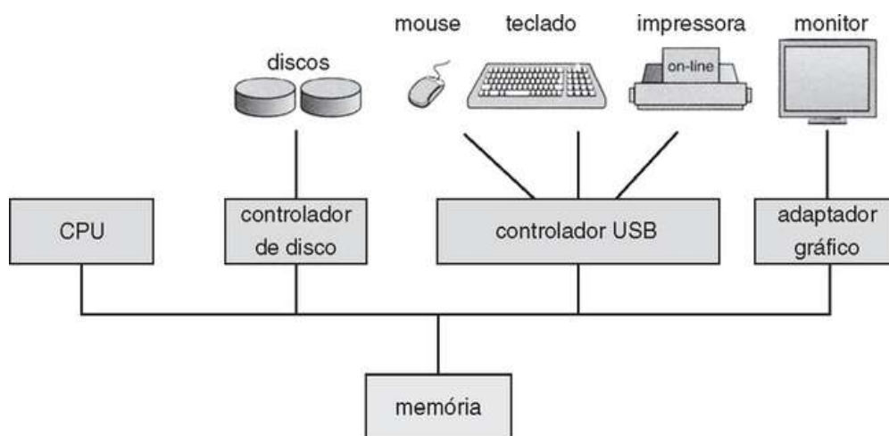
FIGURA 19.1 Organização orientada a barramento.
