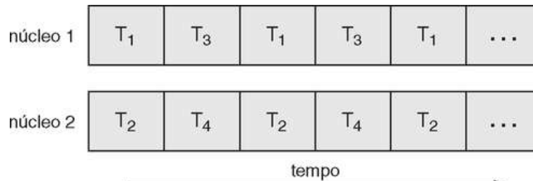
FIGURA 4.4 Execução paralela em um sistema de múltiplos núcleos (multicore).
