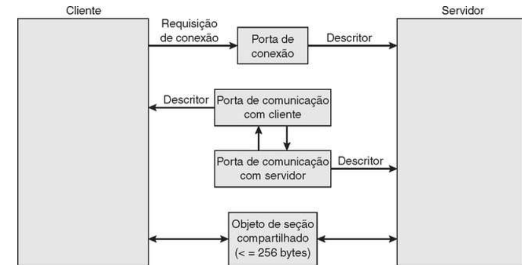
FIGURA 3.24 Chamadas de procedimento local no Windows XP.
