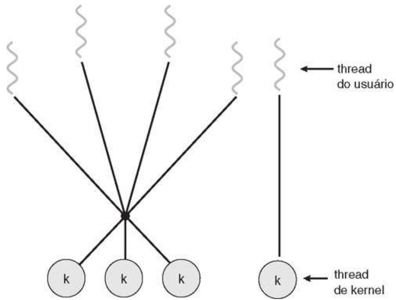
FIGURA 4.8 Modelo de dois níveis (two-level model)
