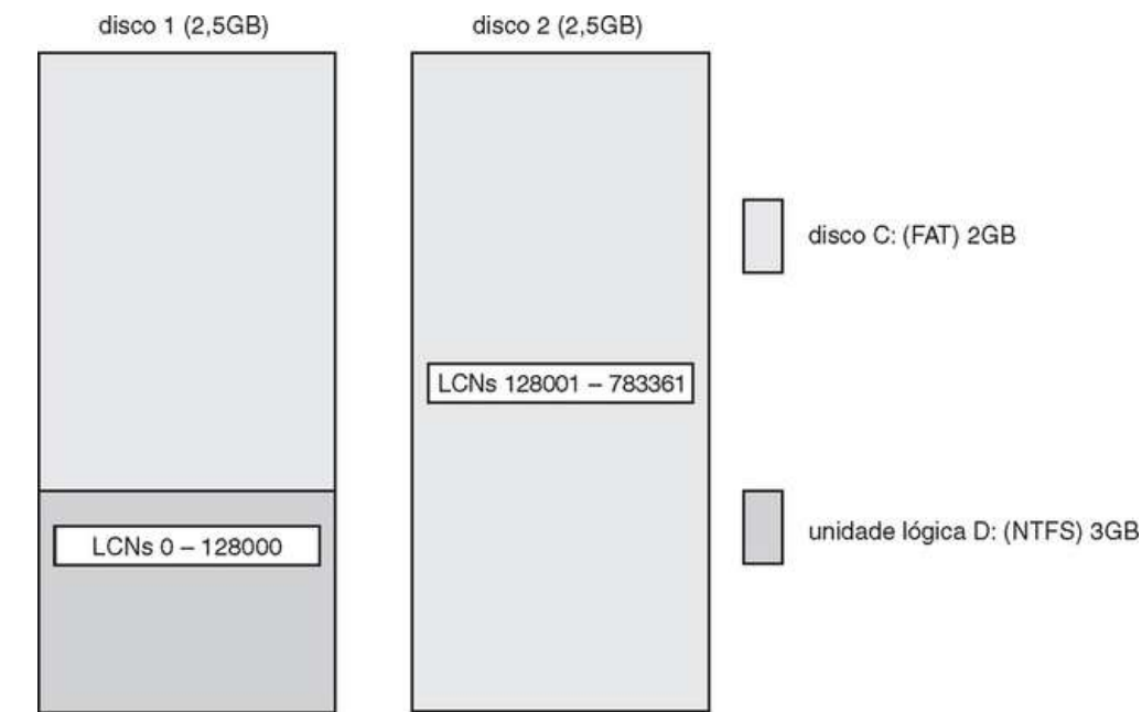
FIGURA 22.7 Conjunto de volumes em duas unidades.
