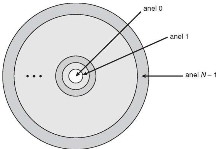
FIGURA 14.2 Estrutura de anel do MULTICS.
