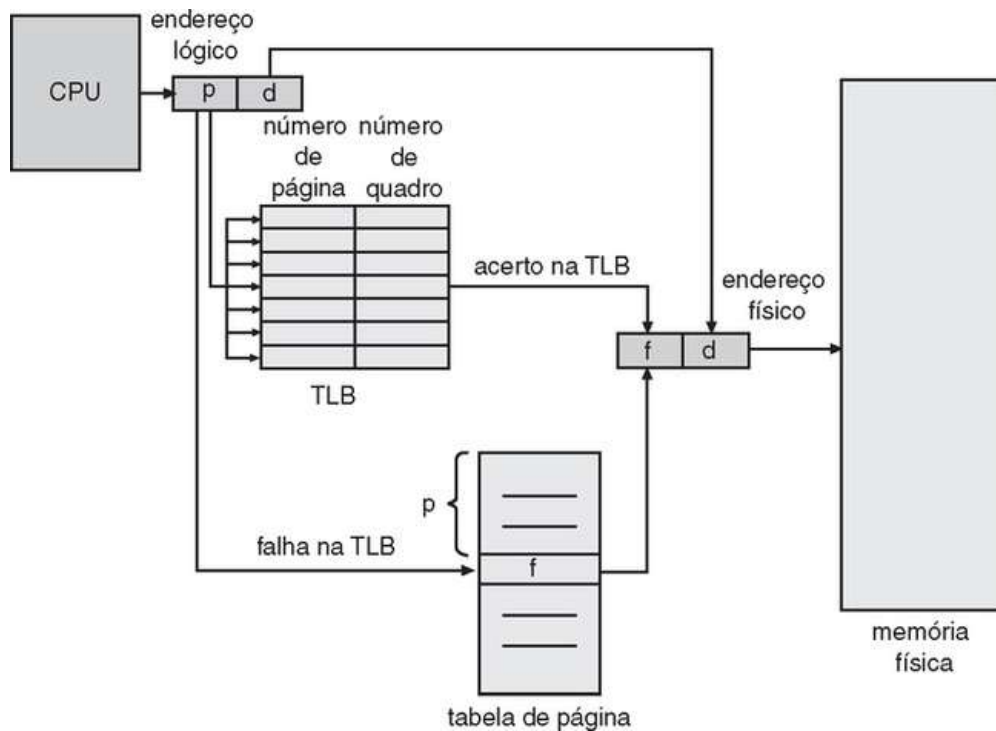
FIGURA 8.11 Hardware de paginação com TLB.
