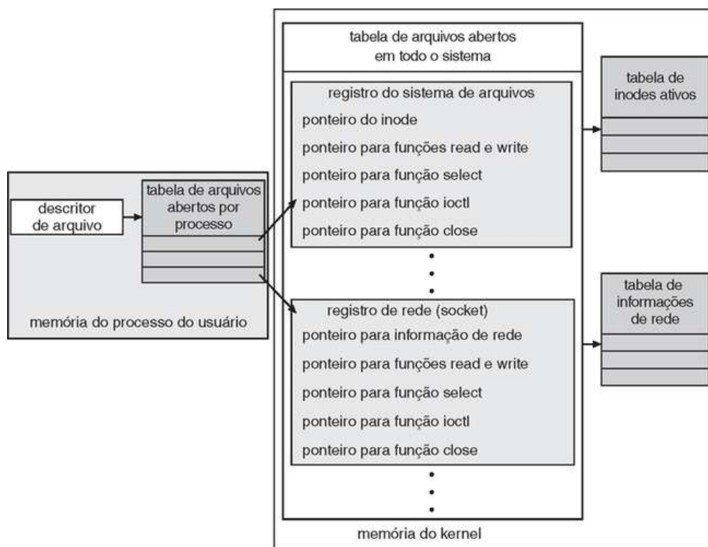
FIGURA 13.12 Estrutura do kernel de E/S do UNIX.
