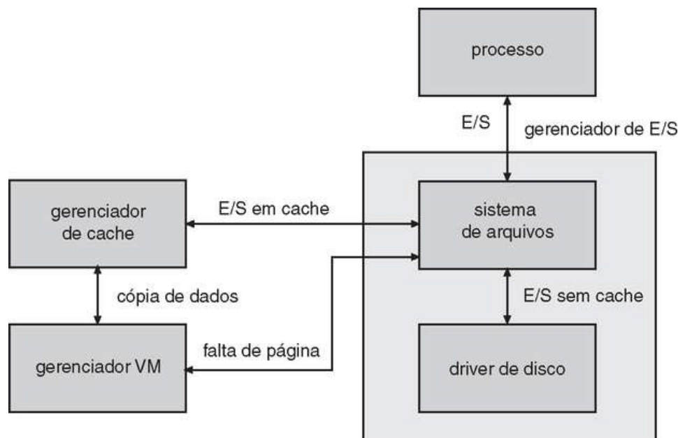
FIGURA 22.6 E/S de arquivo.
