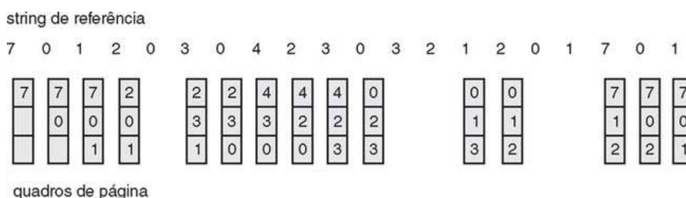
FIGURA 9.12 Algoritmo de substituição de página FIFO.
