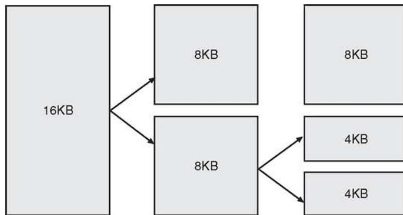
FIGURA 21.6 Dividindo a memória em um sistema buddy.
