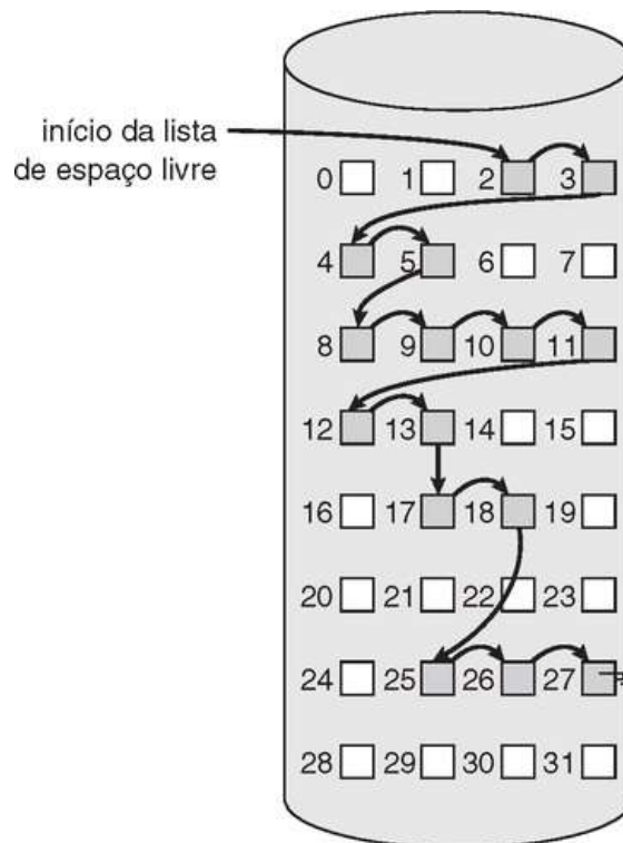
FIGURA 11.10 Lista interligada de espaço livre no disco.
