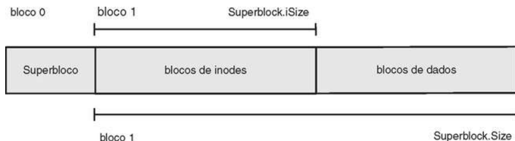
FIGURA 11.18 Estrutura do disco simulado.
