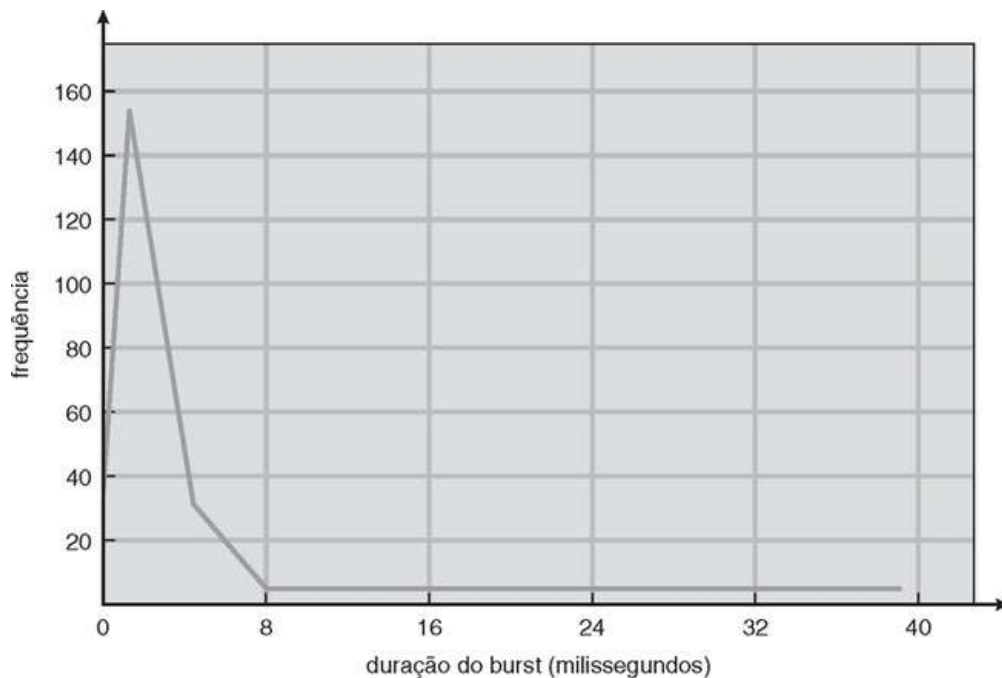
FIGURA 5.2 Histograma dos tempos de burst da CPU.
