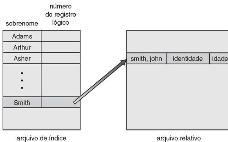
FIGURA 10.5 Exemplo de arquivos de índice e relativo.
