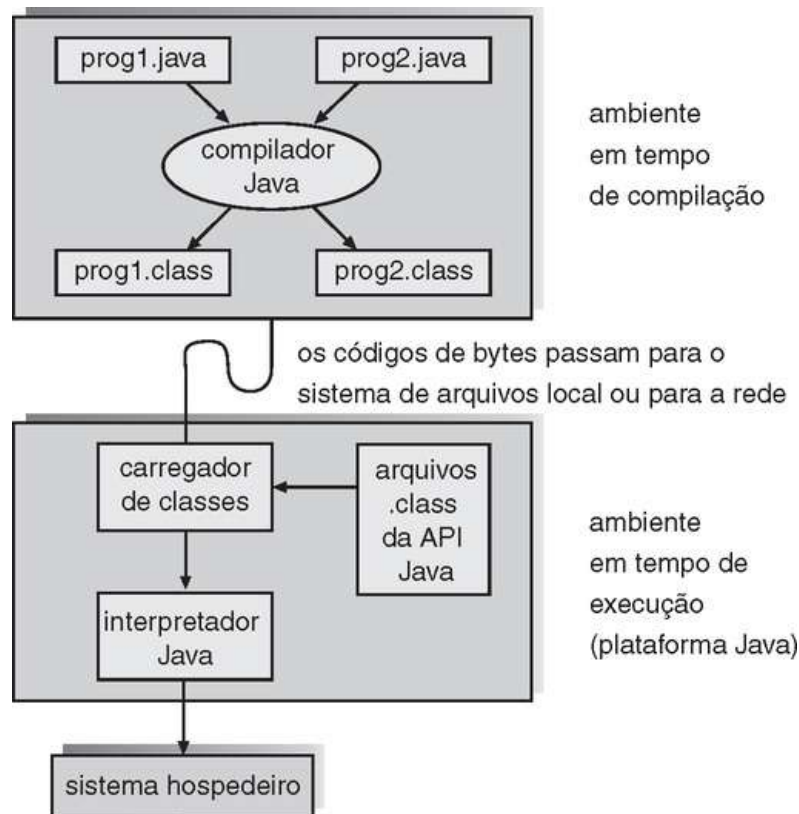
FIGURA 2.21 Ambiente de desenvolvimento Java.
