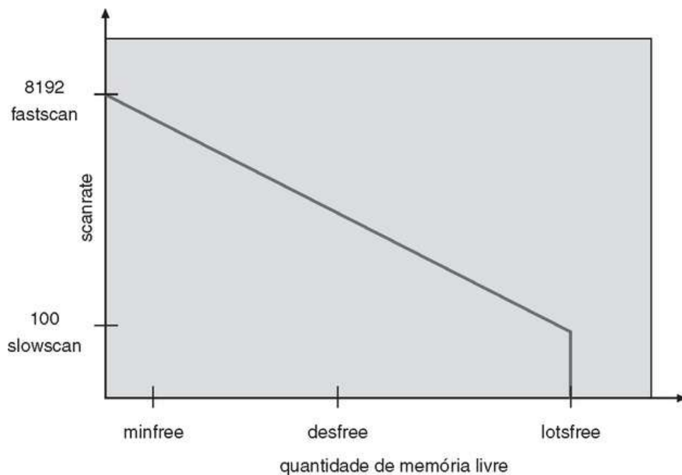
FIGURA 9.29 Verificador de página do Solaris.
