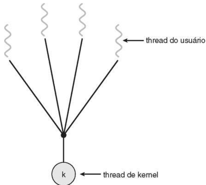
FIGURA 4.5 Modelo muitos para um.
