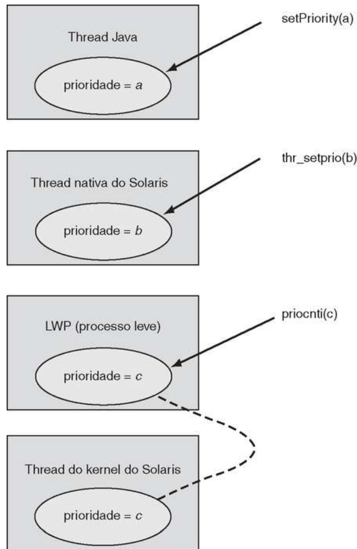
FIGURA 5.19 Threads do usuário são mapeadas para threads do Kernel por meio de um processo leve.
