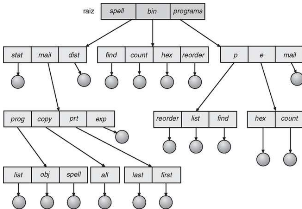
FIGURA 10.10 Estrutura de um diretório estruturado em árvore.
