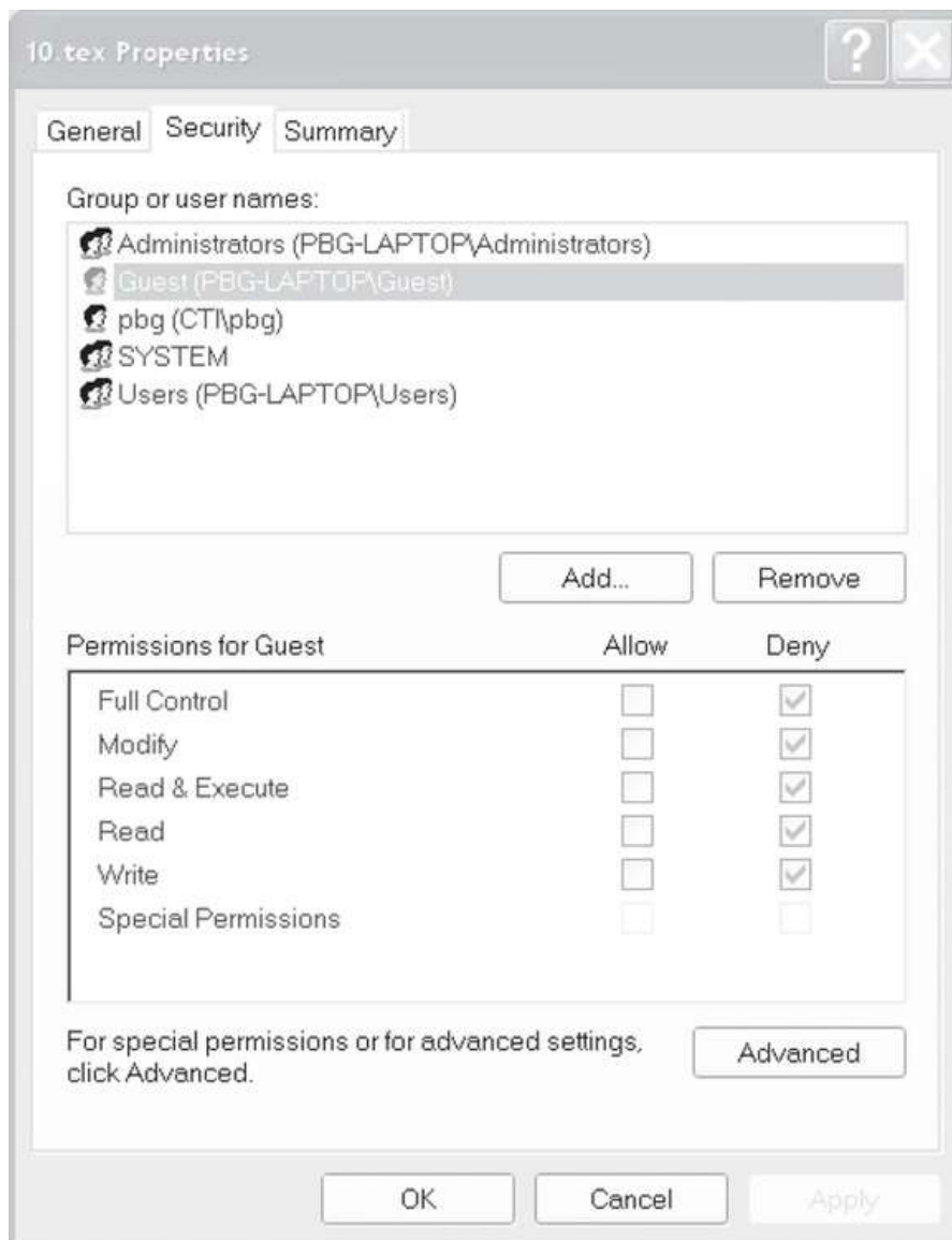
FIGURA 10.15 Gerenciamento da lista de controle de acesso no Windows XP.
