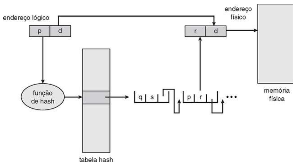
FIGURA 8.16 Tabela de página com hash.
