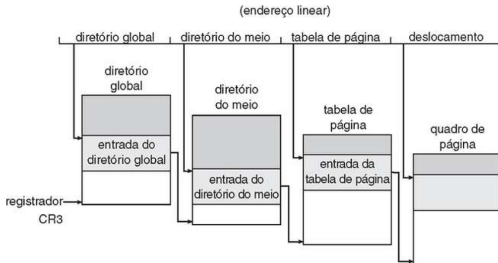
FIGURA 8.24 Paginação em três níveis no Linux.
