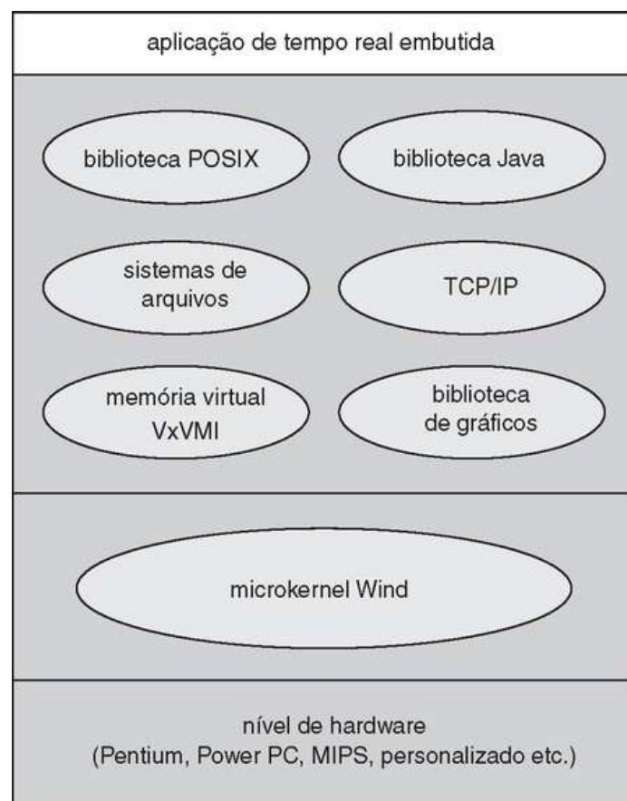
FIGURA 19.12 A organização do VxWorks.
