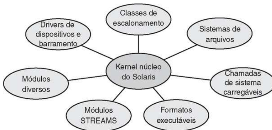
FIGURA 2.15 Módulos carregáveis do Solaris.
