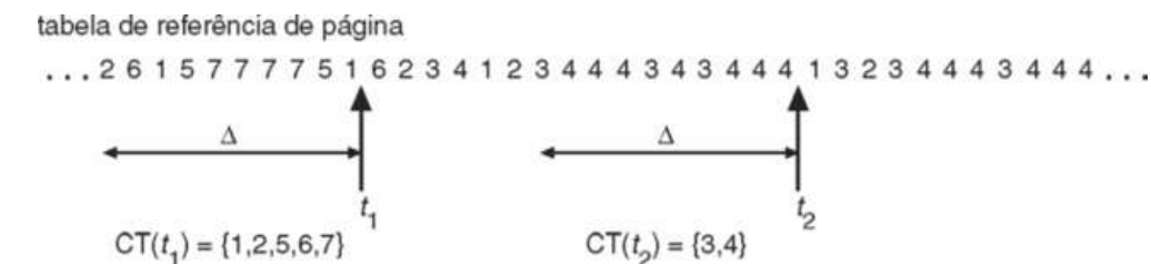
FIGURA 9.20 Modelo do conjunto de trabalho.
