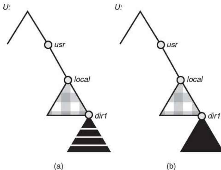
FIGURA 11.14 Montando no NFS. (a) Montagens e (b) montagens em cascata.
