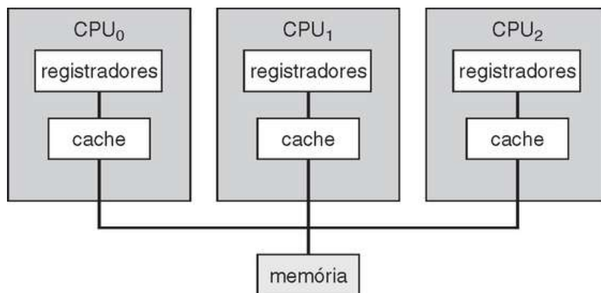
FIGURA 1.6 Arquitetura de multiprocessamento simétrico.
