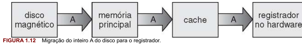
FIGURA 1.12 Migração do inteiro A do disco para o registrador.
