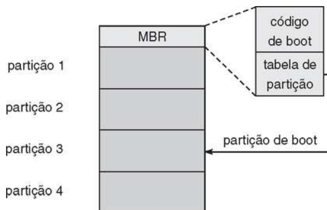
FIGURA 12.9 Booting do disco no Windows 2000.
