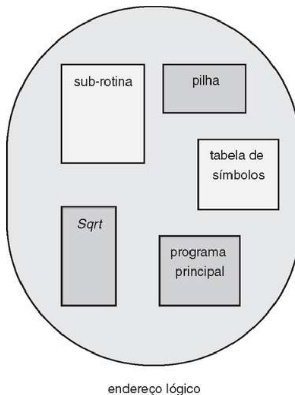
FIGURA 8.18 Visão de um programa pelo usuário.
