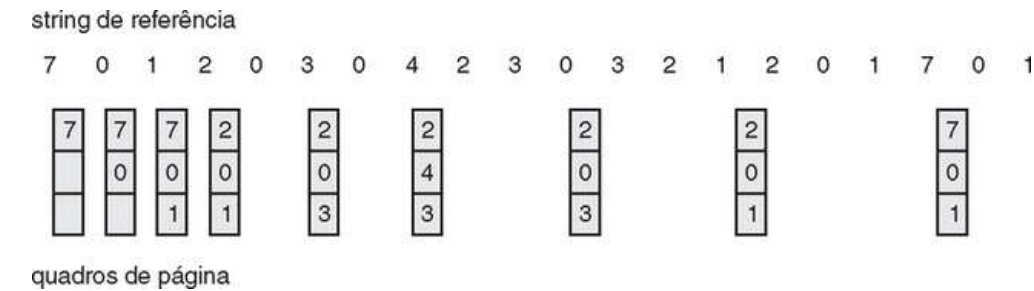
FIGURA 9.14 Algoritmo de substituição de página ótima.
