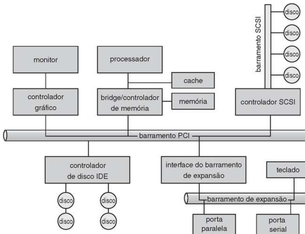
FIGURA 13.1 Uma estrutura típica de barramento do PC.
