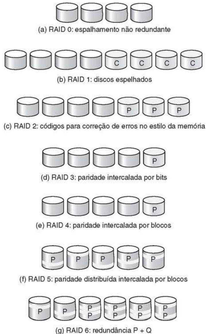
FIGURA 12.11 Níveis de RAID.
