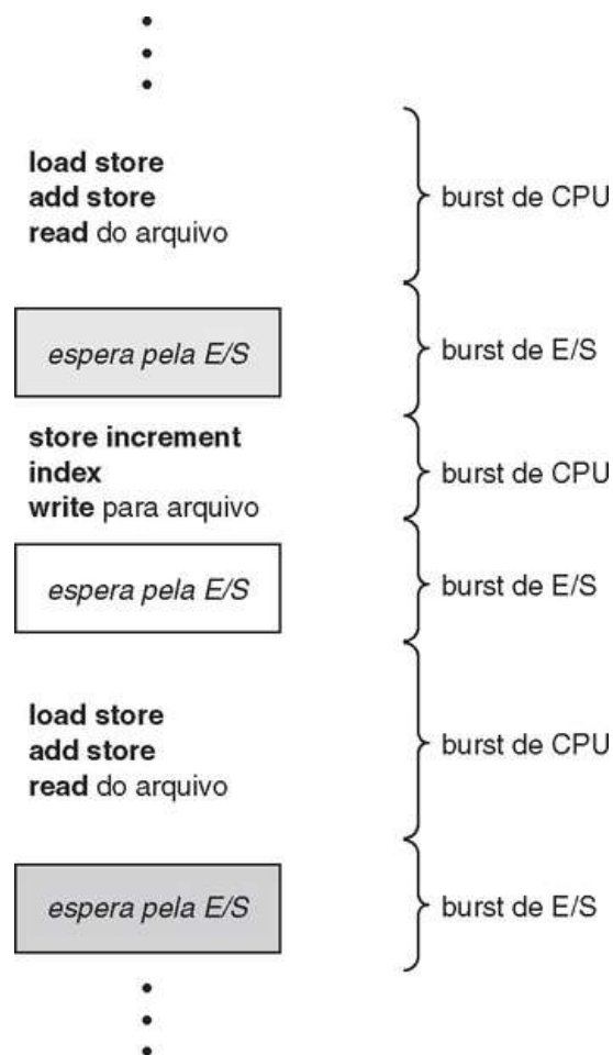
FIGURA 5.1 Alternando a sequência de bursts CPU-E/S.
