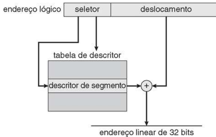
FIGURA 8.22 Segmentação do Intel Pentium.
