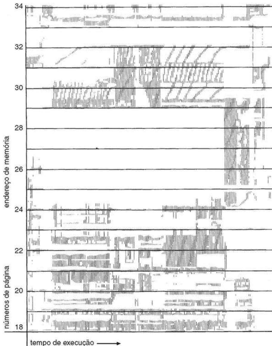
FIGURA 9.19 Localidade em um padrão de referência à memória.
