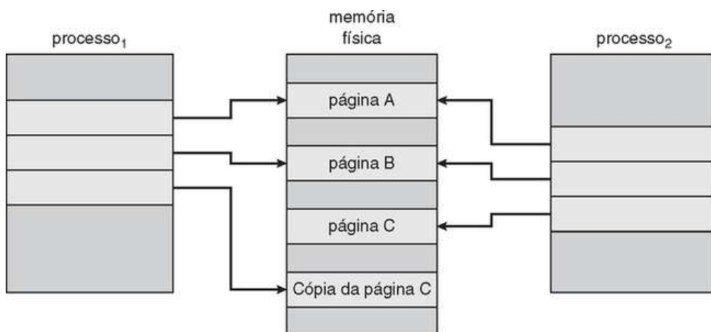
FIGURA 9.8 Depois de o processo 1 modificar a página C.
