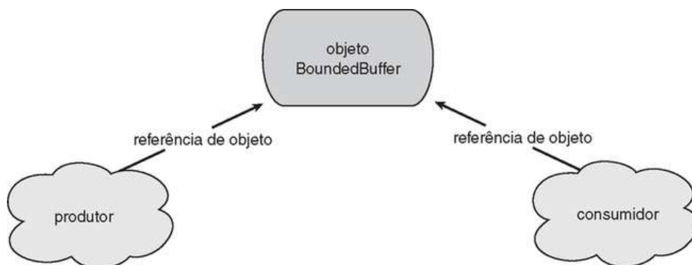
FIGURA 3.19 Simulando a memória compartilhada em Java.
