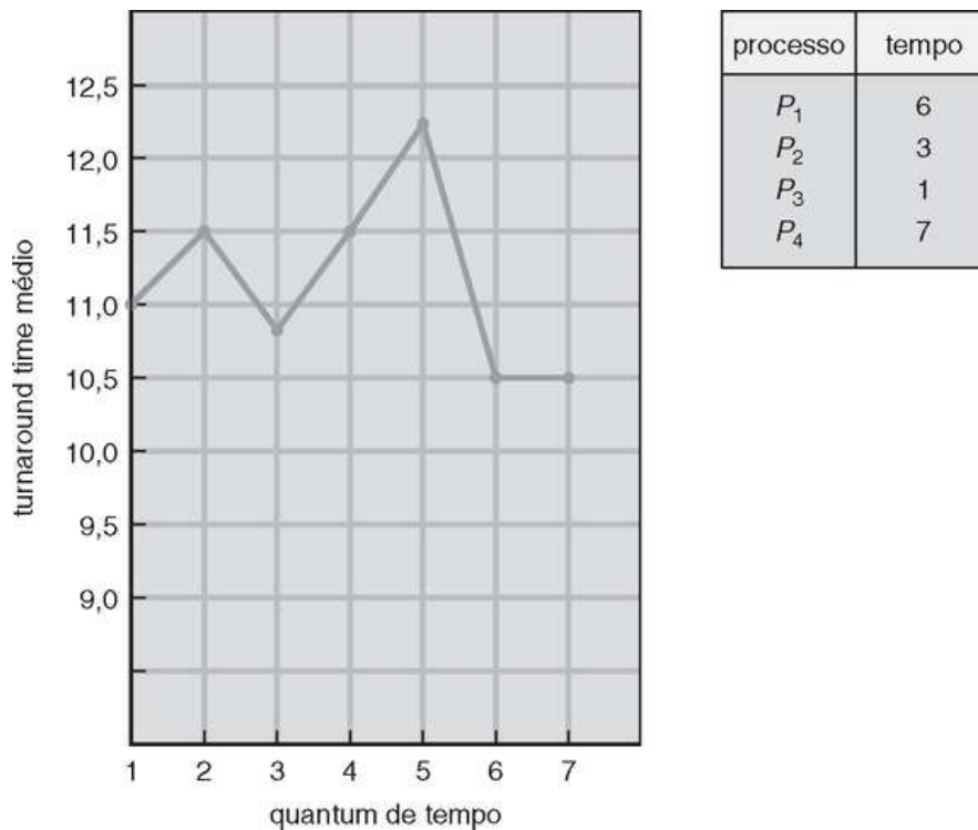
FIGURA 5.5 O modo como o turnaround time varia com o quantum de tempo.
