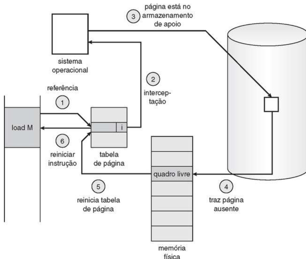
FIGURA 9.6 Etapas no tratamento de uma falha de página (page fault).
