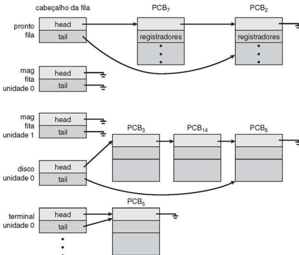
FIGURA 3.6 A fila de prontos e diversas filas de dispositivo de E/S.
