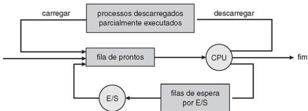
FIGURA 3.8 Acréscimo do escalonamento de meio-termo para o diagrama de enfileiramento.
