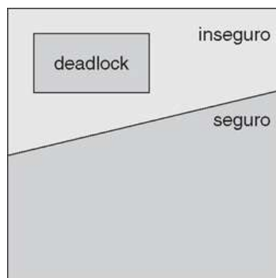
FIGURA 7.8 Espaço dos estados seguro, inseguro e com deadlock.
