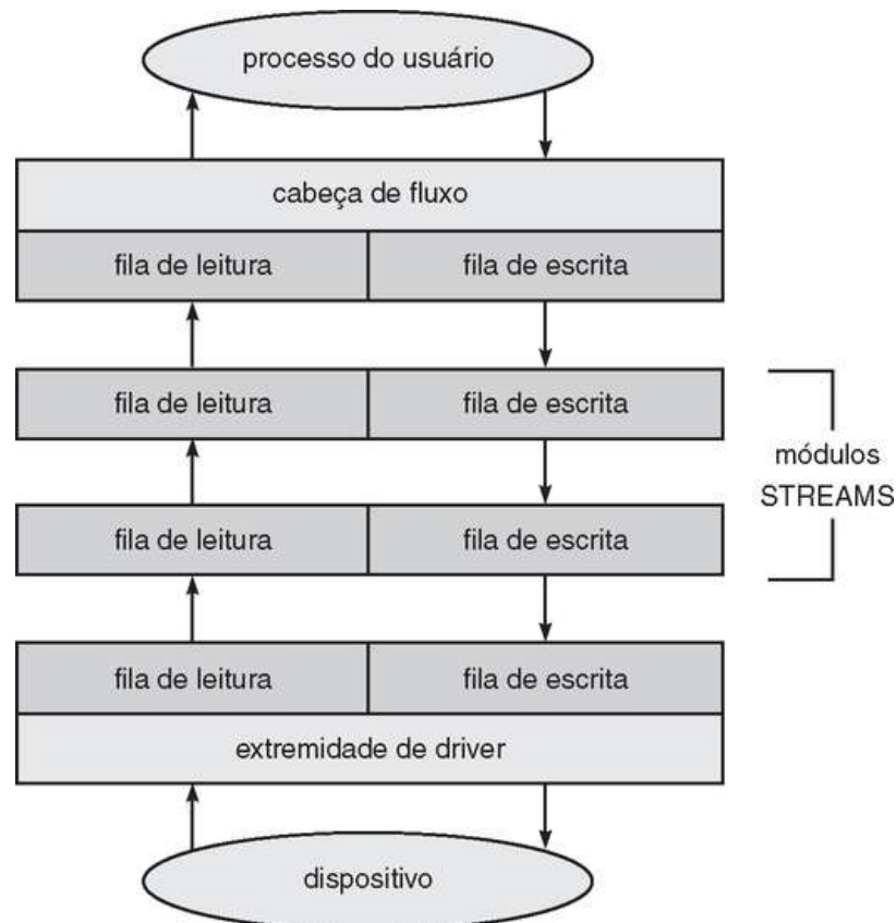
FIGURA 13.14 A estrutura STREAMS.
