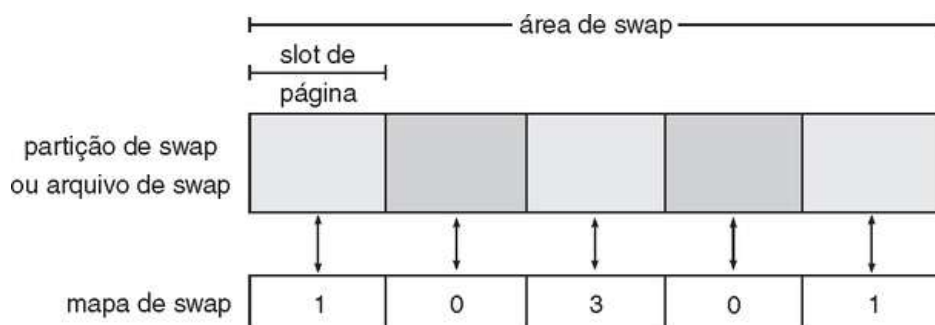
FIGURA 12.10 As estruturas de dados para o swapping nos sistemas Linux.
