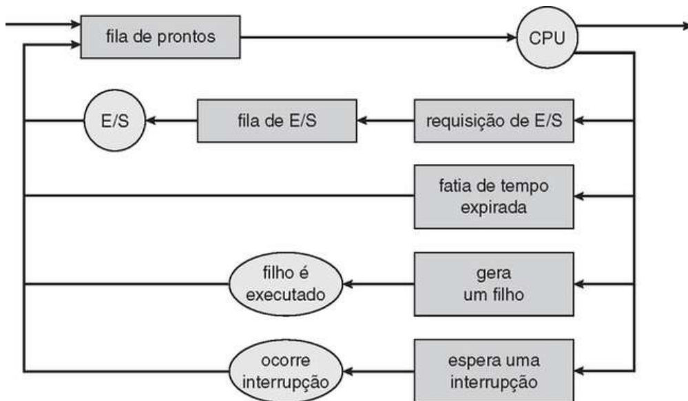
FIGURA 3.7 A representação do diagrama de fila do escalonamento de processos.
