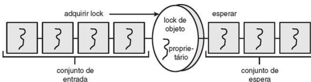
FIGURA 6.30 Conjuntos de entrada e espera
