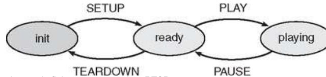
FIGURA 20.4 Máquina de estado finito representando o RTSP.
