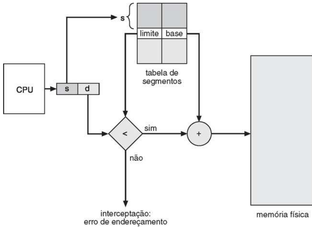
FIGURA 8.19 Hardware de segmentação.
