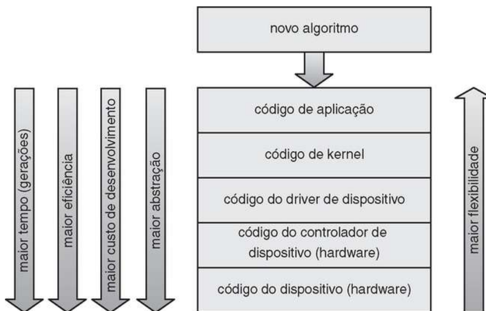
FIGURA 13.16 Progressão da funcionalidade do dispositivo.
