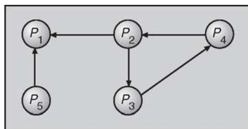
FIGURA 18.4 Grafo de espera global para a Figura 18.3 .
