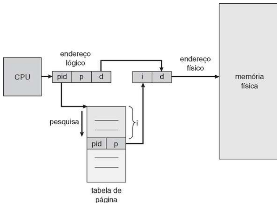
FIGURA 8.17 Tabela de página invertida.
