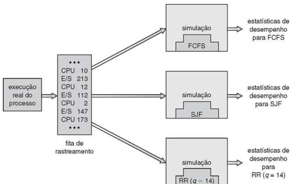
FIGURA 5.21 Avaliação dos escalonadores de CPU pela simulação.
