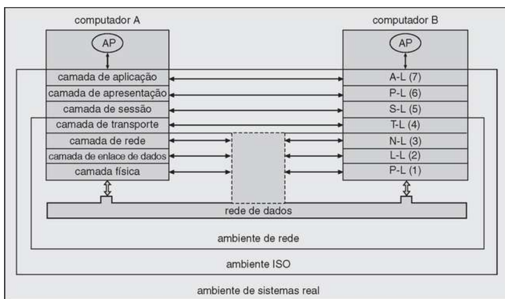
FIGURA 16.6 Dois computadores se comunicando por meio do modelo de rede ISO.
