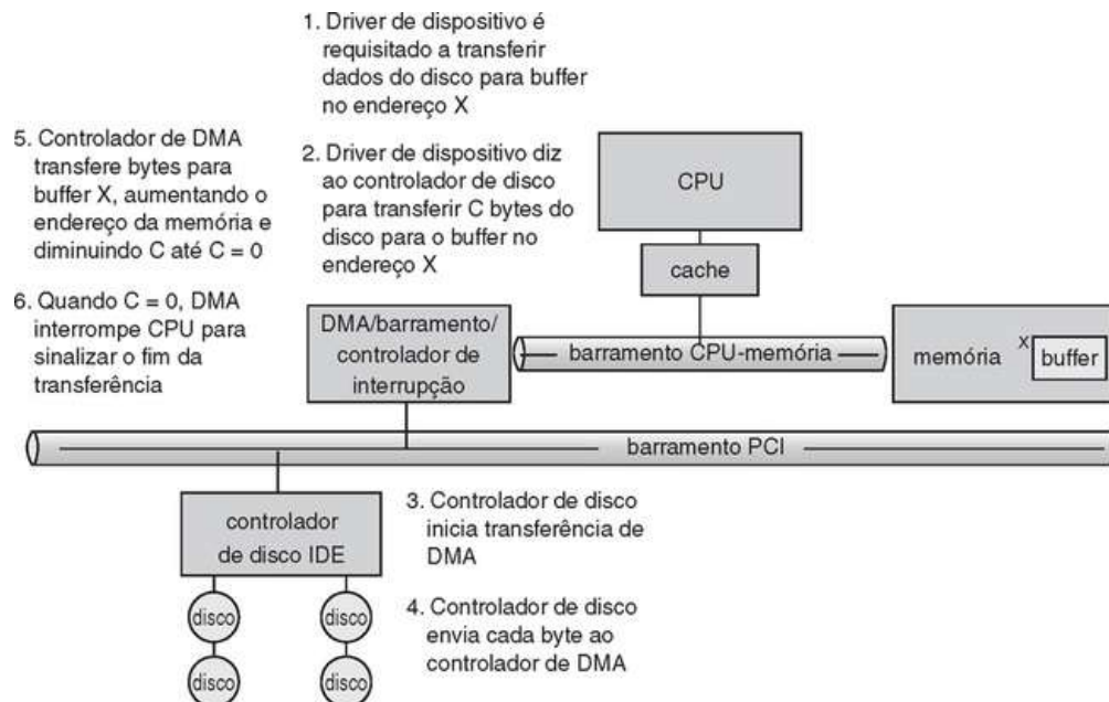
FIGURA 13.5 Etapas em uma transferência de DMA.
