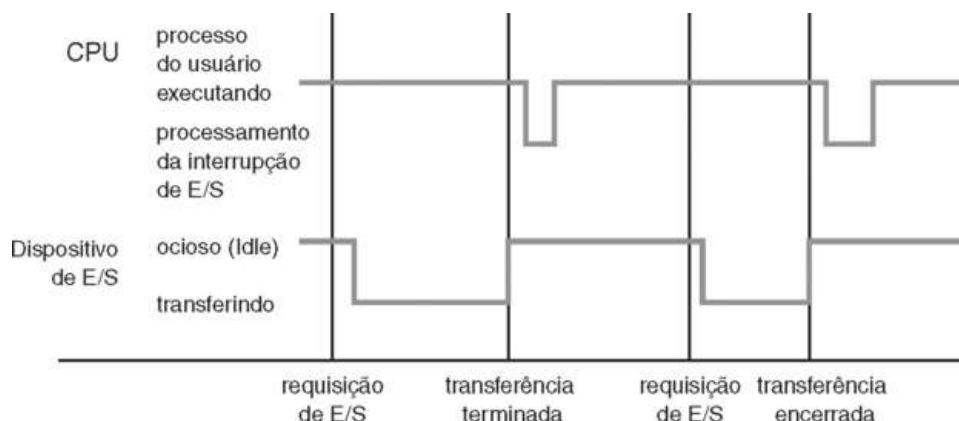
FIGURA 1.3 Linha de tempo da interrupção para um único processo efetuando uma saída.
