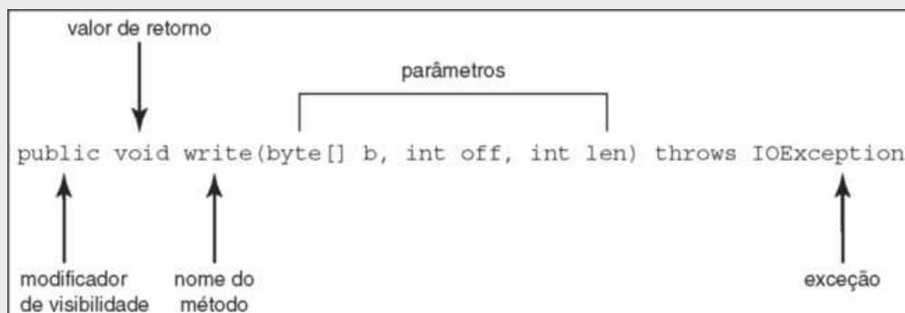
FIGURA 2.5 API para o método write() .
