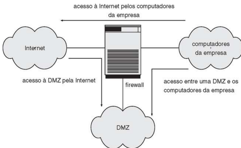
FIGURA 15.10 Separação de domínio via firewall.
