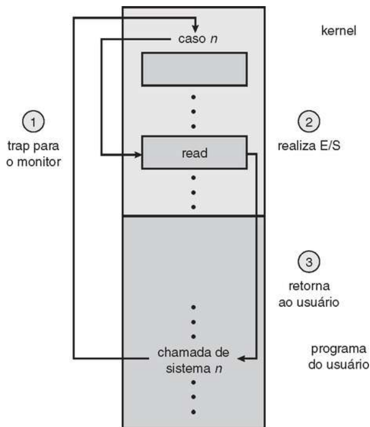
FIGURA 13.11 Uso de uma chamada de sistema para realizar E/S.
