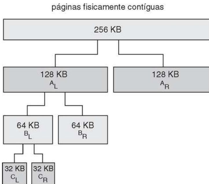
FIGURA 9.26 Alocação de sistema buddy.
