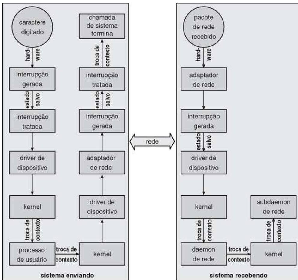
FIGURA 13.15 Comunicações entre computadores.
