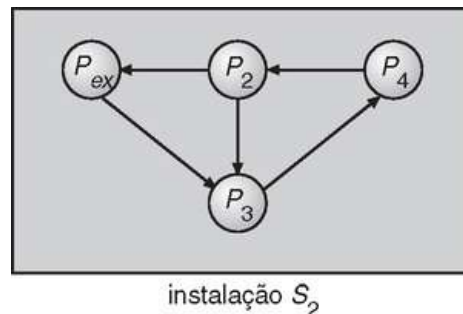
FIGURA 18.7 Grafo de espera local aumentado na instalação S_2 da Figura 18.6.
