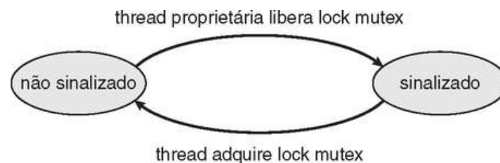
FIGURA 6.39 Objeto despachante mutex
