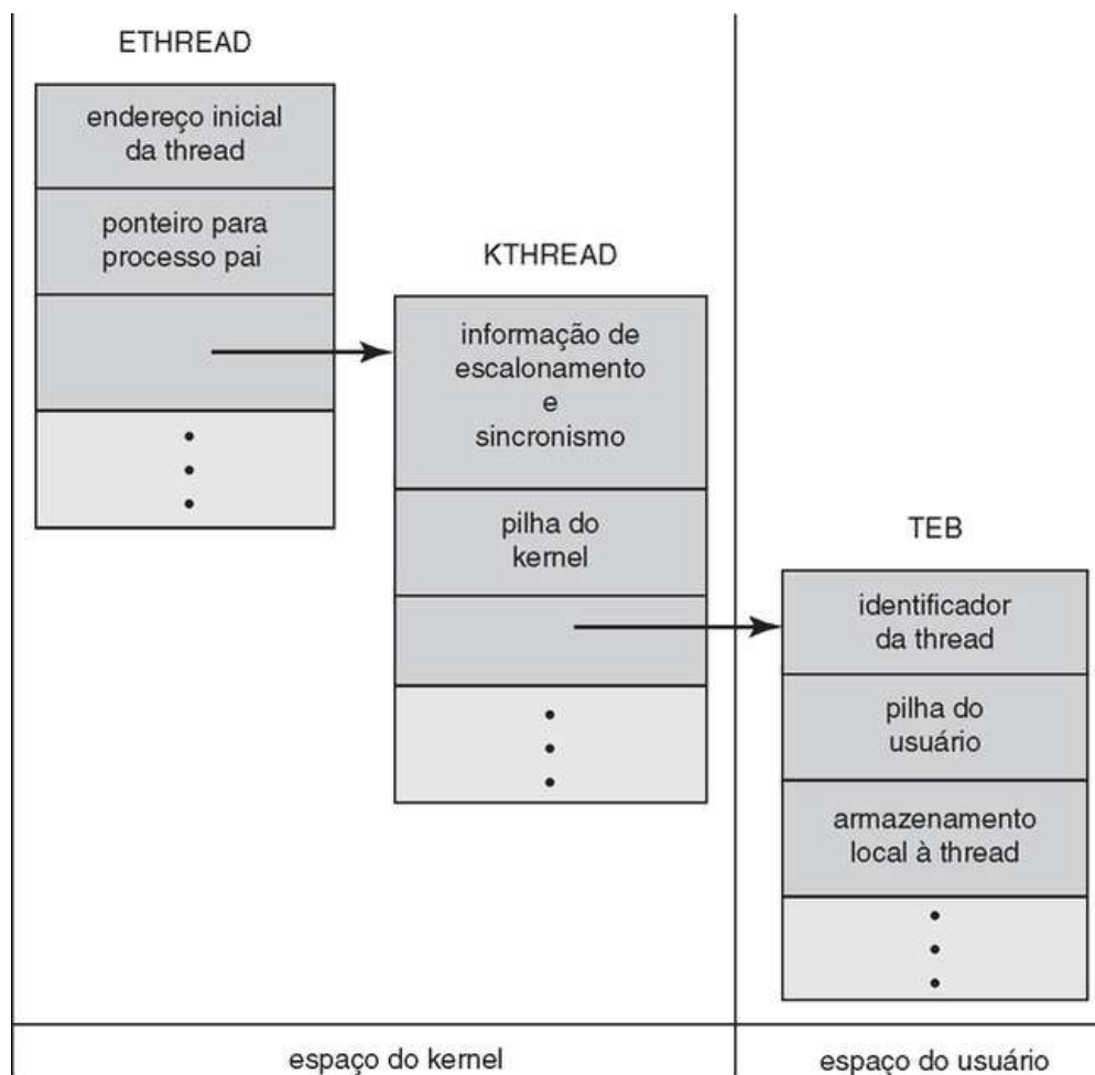
FIGURA 4.21 Estruturas de dados de uma thread no Windows XP.
