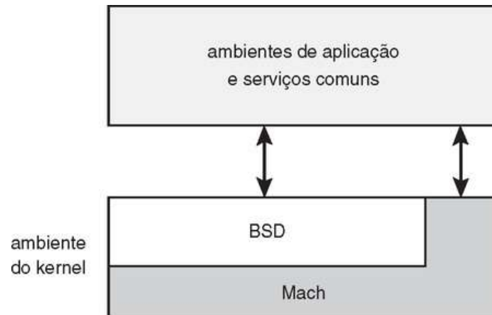
FIGURA 2.16 A estrutura do Mac OS X.
