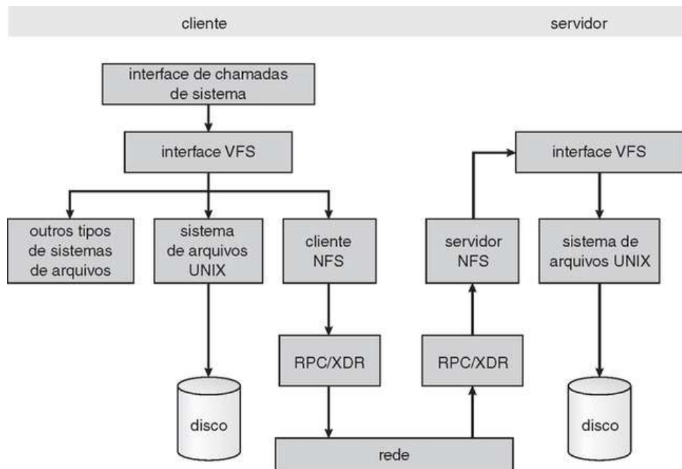
FIGURA 11.15 Visão esquemática da arquitetura do NFS.
