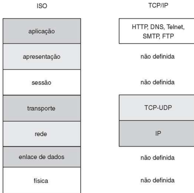
FIGURA 16.9 As pilhas de protocolo ISO e TCP/IP.
