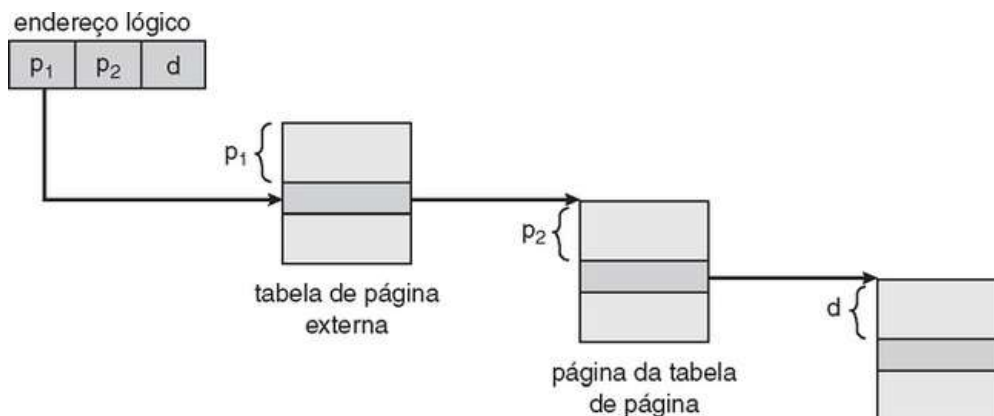
FIGURA 8.15 Tradução de endereço para uma arquitetura de página de 32 bits em dois níveis.
