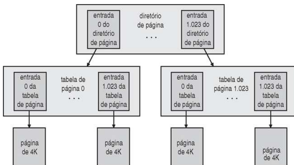
FIGURA 22.3 Layout da tabela de página.
