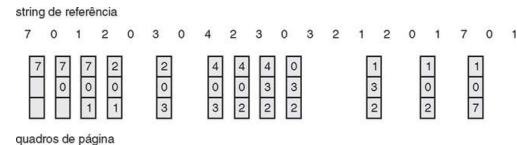
FIGURA 9.15 Algoritmo de substituição de página LRU.
