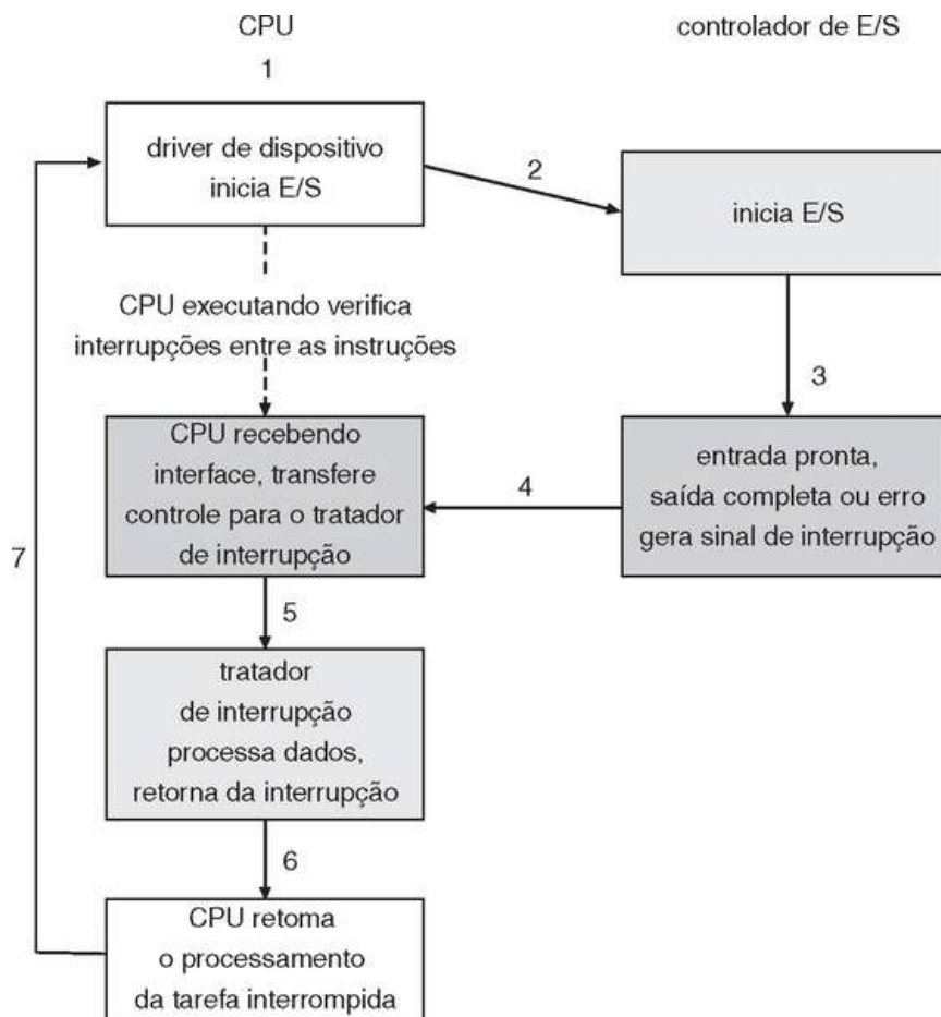
FIGURA 13.3 Ciclo de E/S controlado por interrupção.
