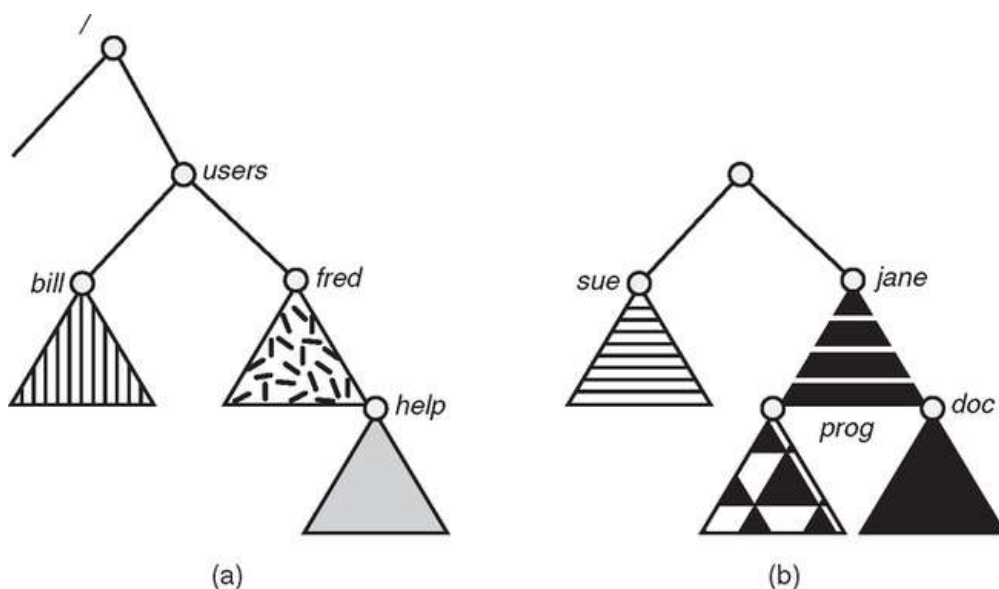
FIGURA 10.13 Sistema de arquivos. (a) Existente e (b) volume não montado.
