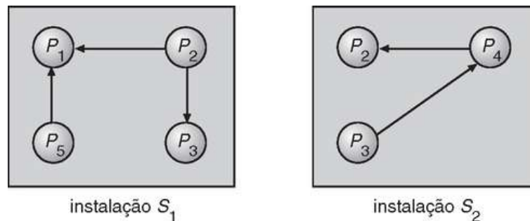
FIGURA 18.3 Dois grafos de espera locais.
