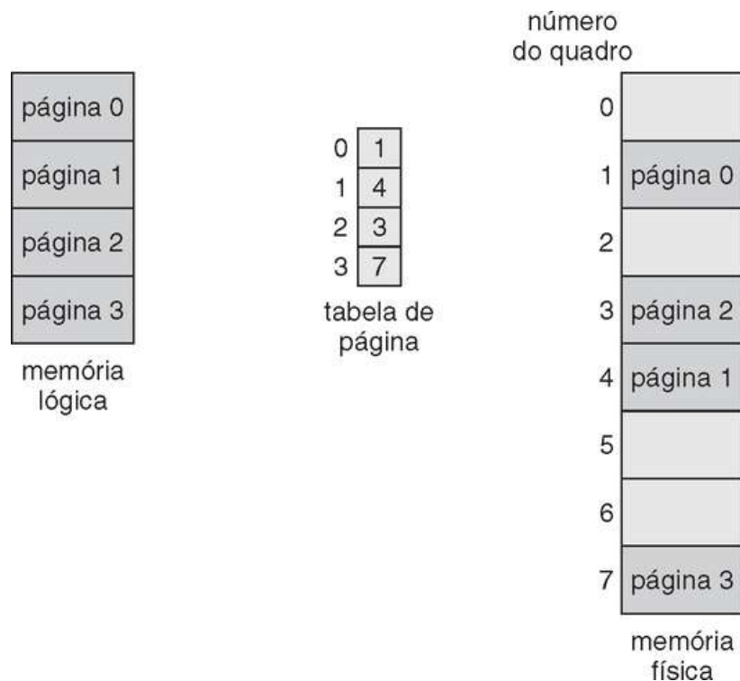
FIGURA 8.8 Modelo de paginação da memória lógica e física.
