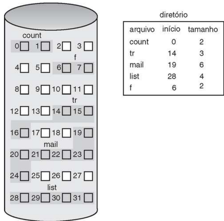
FIGURA 11.5 Alocação contígua do espaço em disco.
