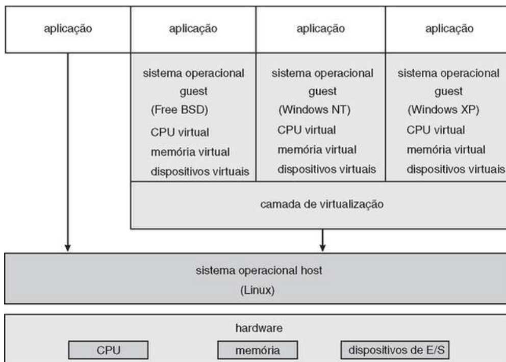
FIGURA 2.18 Arquitetura do VMware.
