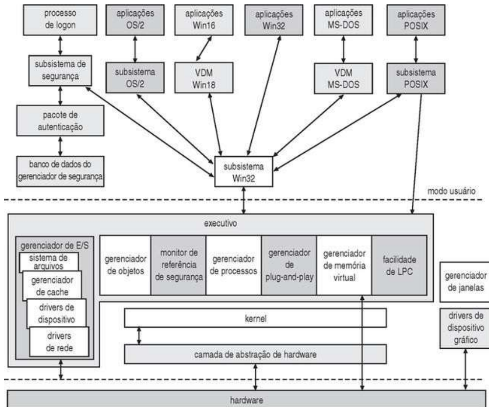
FIGURA 22.1 Diagrama em blocos do Windows XP.
