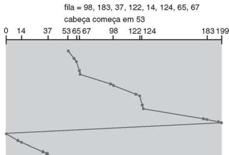
FIGURA 12.7 Escalonamento de disco C-SCAN.
