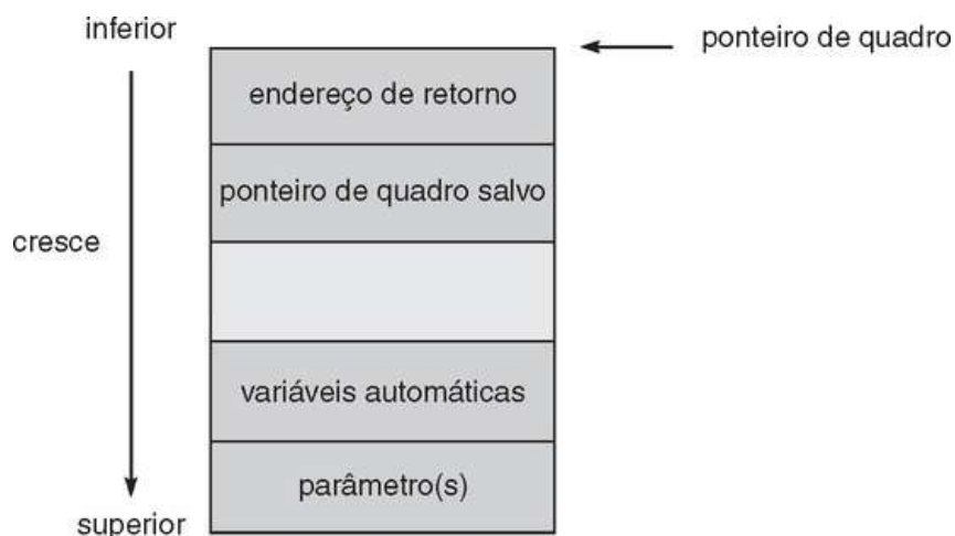
FIGURA 15.3 O layout de um quadro de pilha típico.
