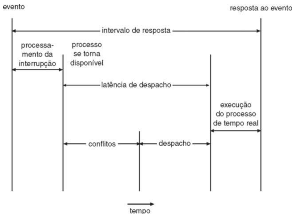
FIGURA 19.5 Latência de despacho.
