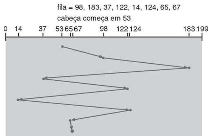
FIGURA 12.4 Escalonamento de disco FCFS.
