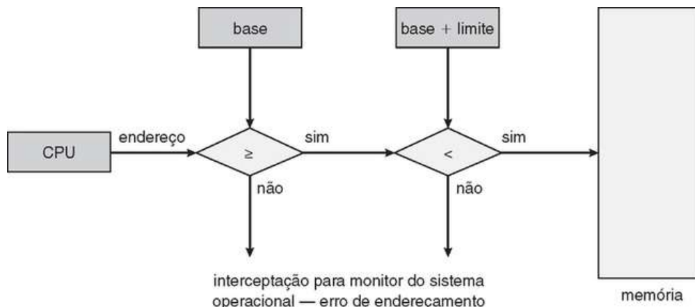
FIGURA 8.2 Proteção de endereço de hardware com registradores de base e limite.
