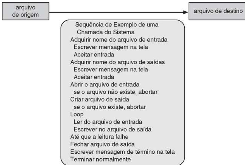
FIGURA 2.4 Exemplo de como são usadas as chamadas de sistema.
