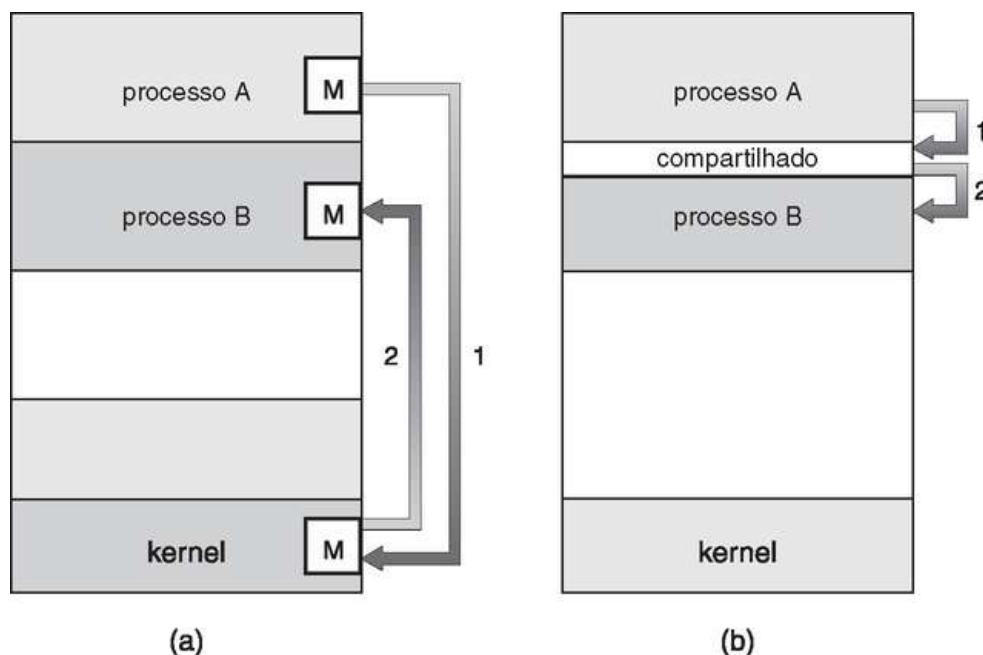
FIGURA 3.14 Modelos de comunicações. (a) Troca de mensagem e (b) memória compartilhada.
