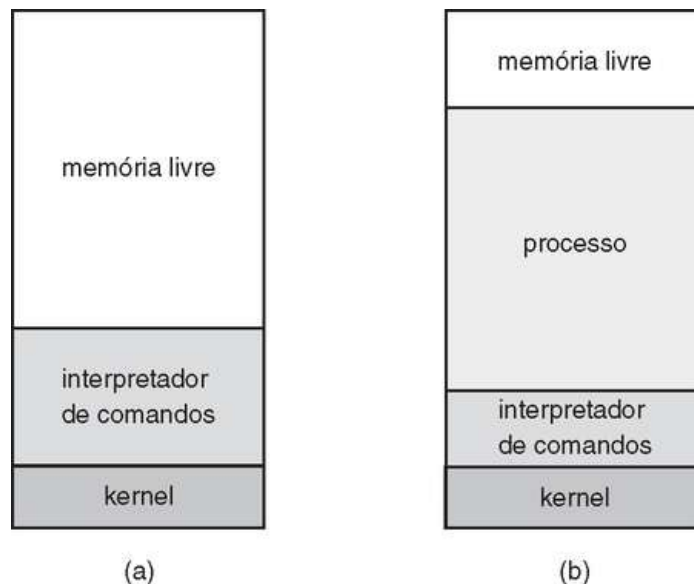
FIGURA 2.10 Execução do MS-DOS: (a) no boot do sistema e (b) executando um programa.
