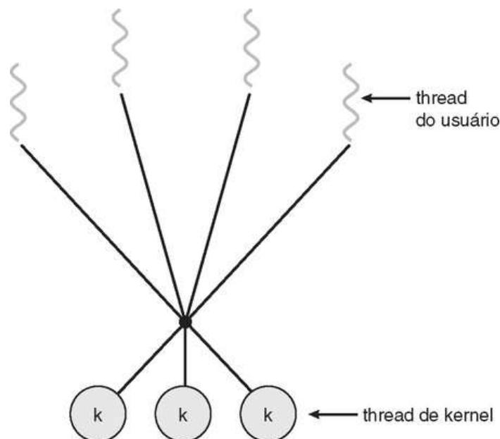
FIGURA 4.7 Modelo muitos para muitos.
