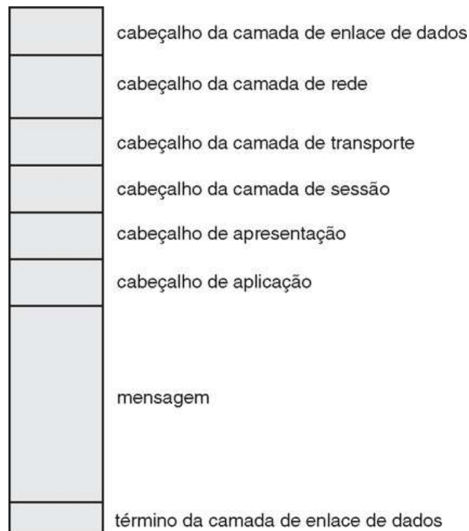
FIGURA 16.8 Uma mensagem de rede ISO.
