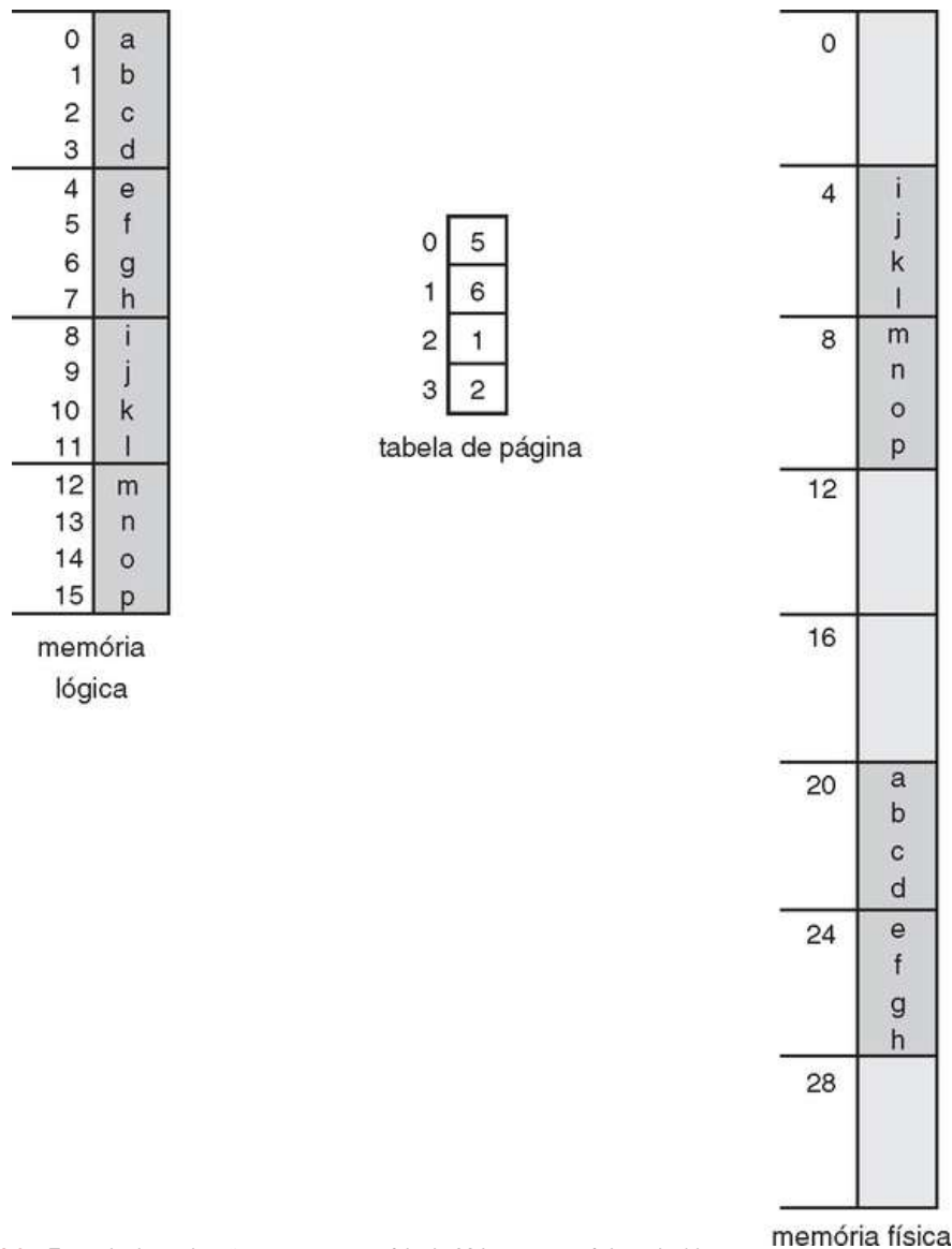
FIGURA 8.9 Exemplo de paginação para uma memória de 32 bytes com páginas de 4 bytes.
