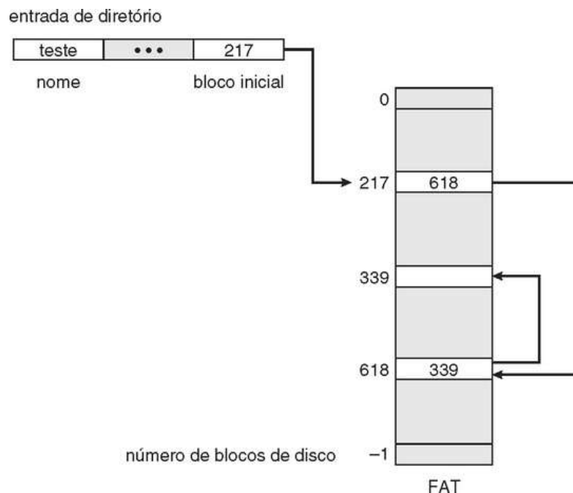
FIGURA 11.7 Tabela de alocação de arquivo.
