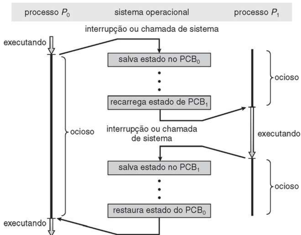
FIGURA 3.4 Troca de CPU de um processo para outro.
