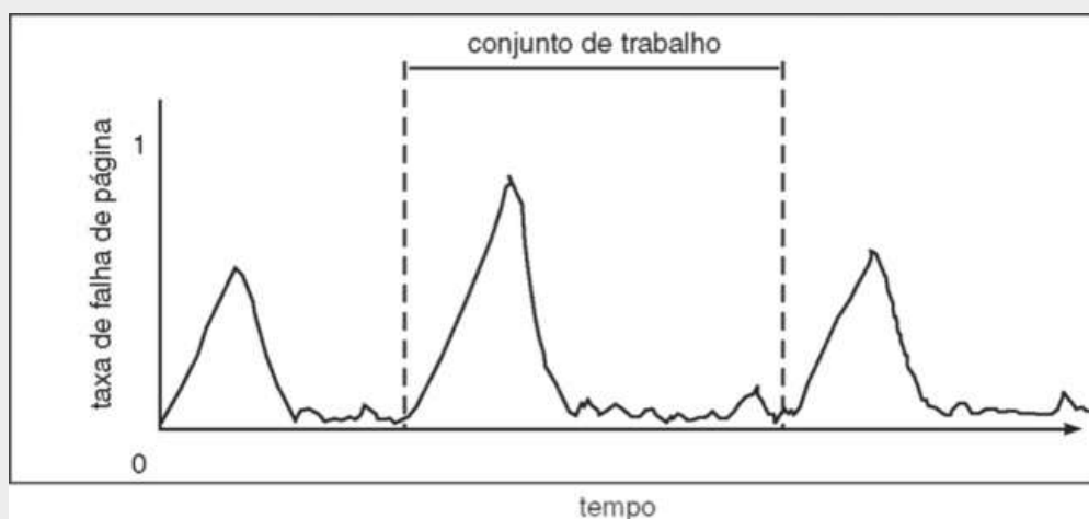
FIGURA 9.22 Taxa de falha de página com o passar do tempo.
