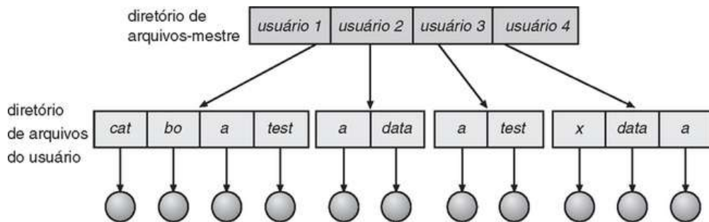
FIGURA 10.9 Estrutura de diretório de dois níveis.
