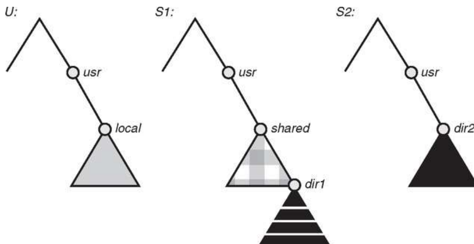
FIGURA 11.13 Três sistemas de arquivos independentes.
