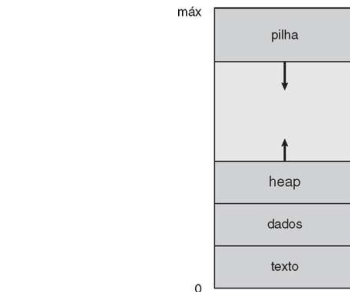
FIGURA 3.1 Processo na memória.
