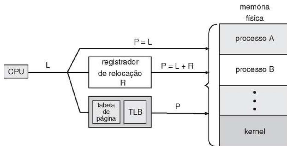
FIGURA 19.2 Tradução de endereços nos sistemas de tempo real.
