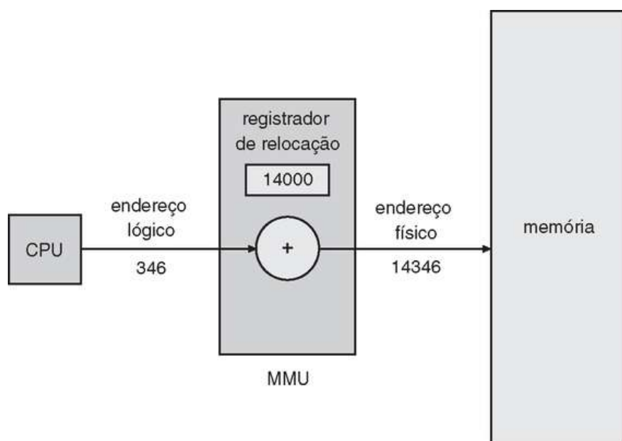
FIGURA 8.4 Relocação dinâmica usando um registrador de relocação.
