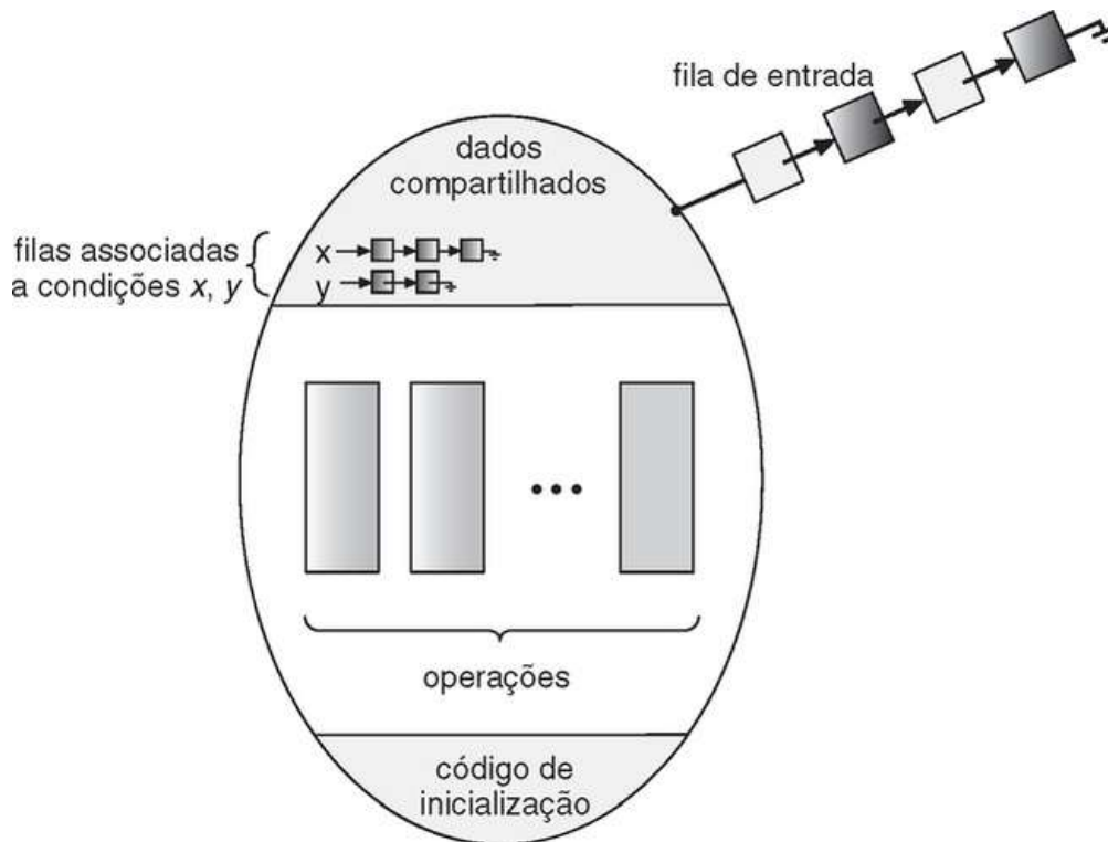
FIGURA 6.25 Monitor com variáveis de condição
