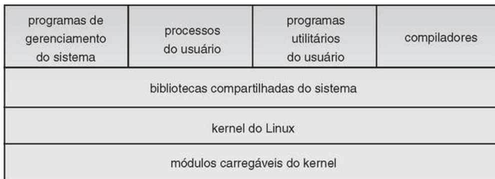
FIGURA 21.1 Componentes do sistema Linux.
