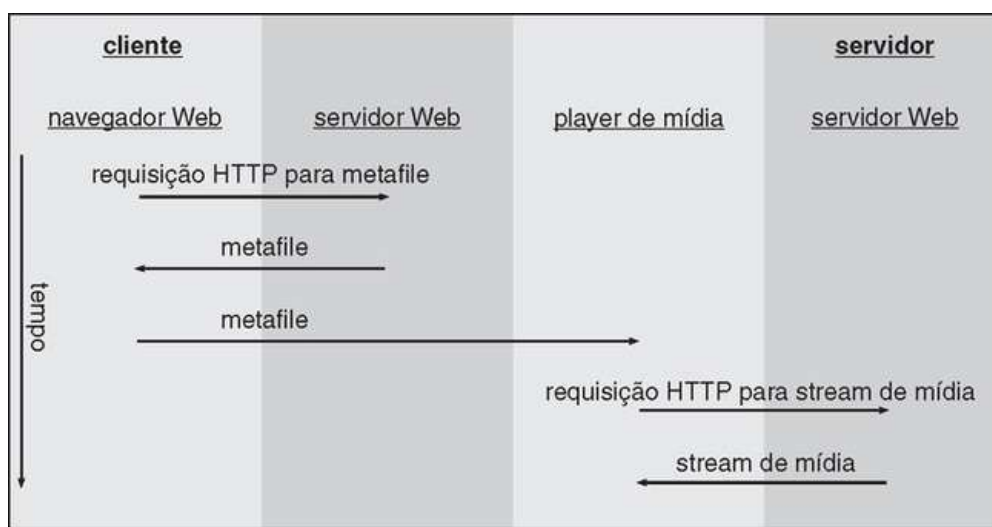
FIGURA 20.2 Mídia streaming de um servidor Web convencional.
