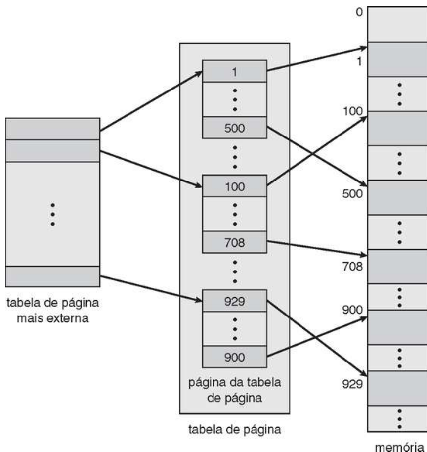
FIGURA 8.14 Um esquema de tabela de página de dois níveis.
