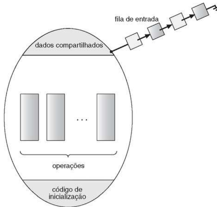
FIGURA 6.24 Visão esquemática de um monitor
