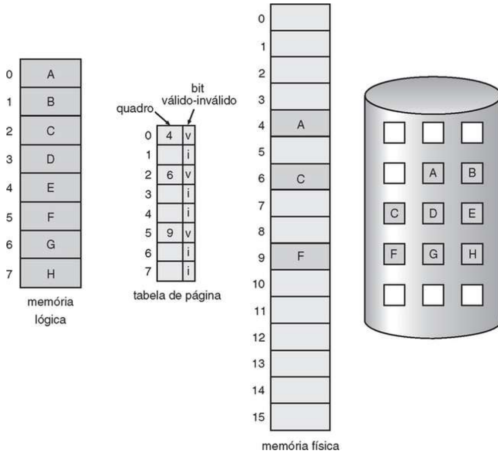
FIGURA 9.5 Tabela de página quando algumas páginas não estão na memória principal.
