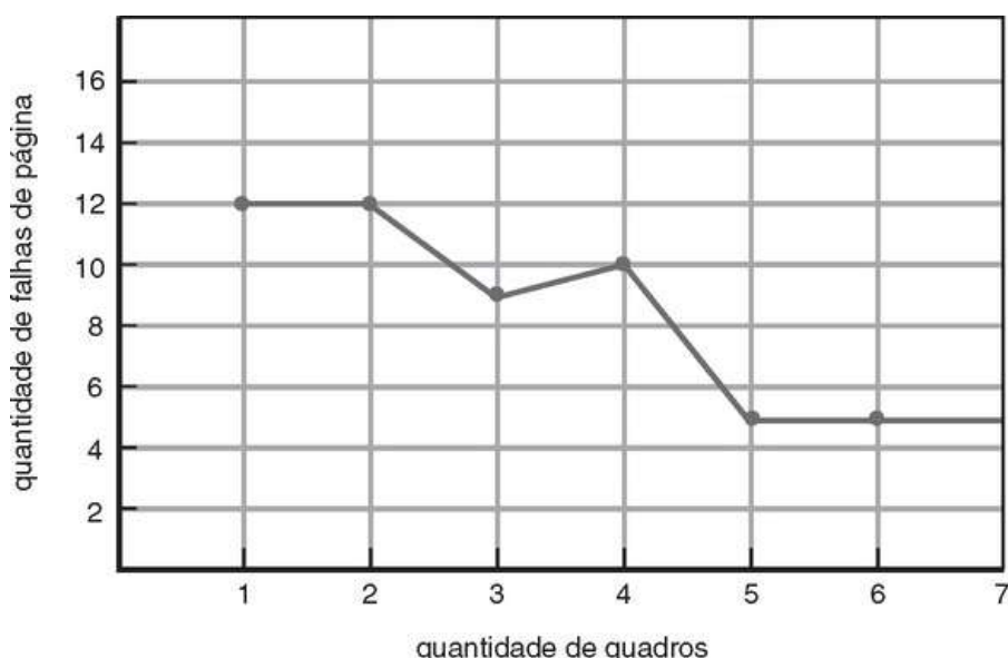
FIGURA 9.13 Curva de falha de página para a substituição FIFO sobre uma string de referência.
