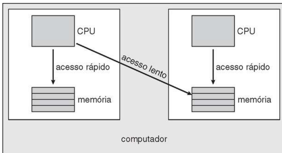
FIGURA 5.9 NUMA e escalonamento de CPU.
