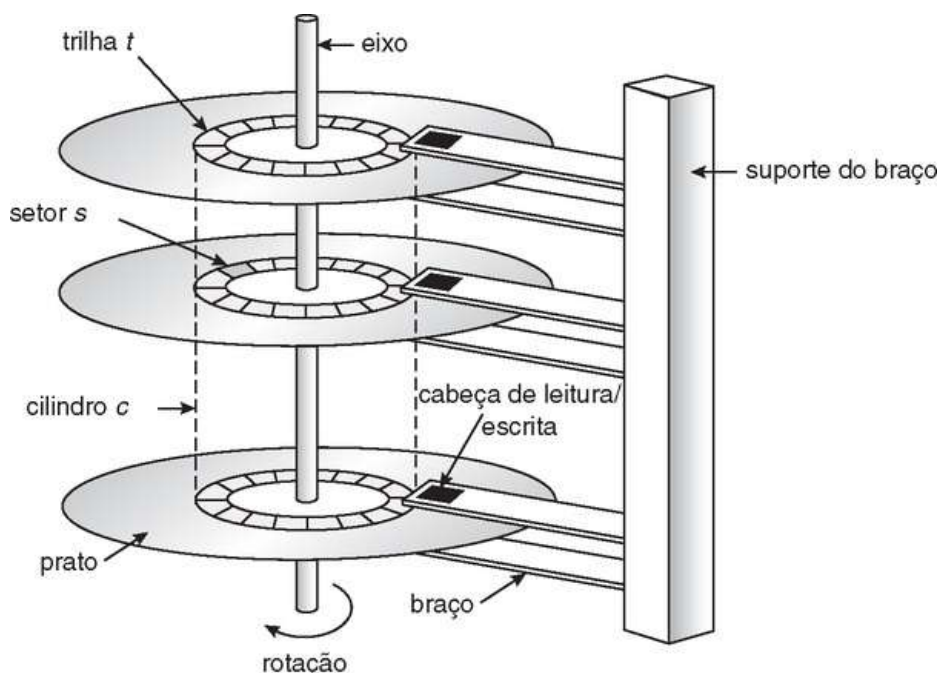
FIGURA 12.1 Mecanismo de disco com cabeça móvel.
