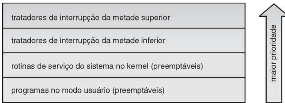
FIGURA 21.4 Níveis de proteção de interrupção.
