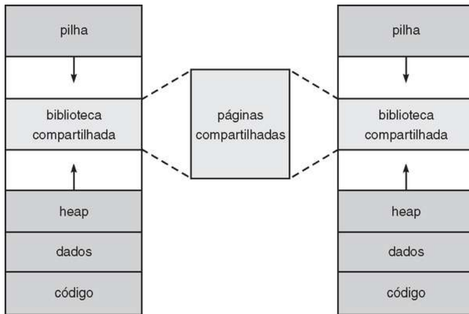
FIGURA 9.3 Biblioteca compartilhada usando memória virtual.
