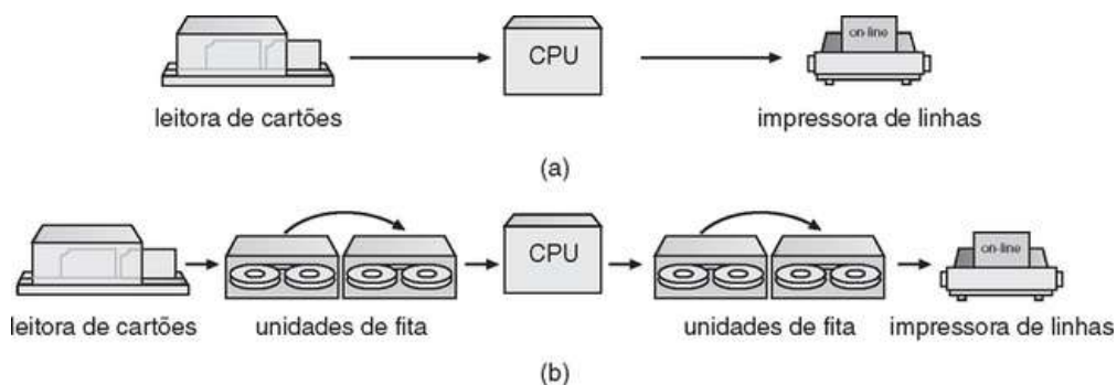
FIGURA 23.4 Operação de dispositivos de E/S (a) on-line e (b) off-line.
