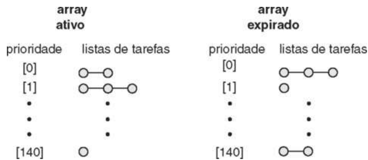
FIGURA 21.3 Listas de tarefas indexadas de acordo com a prioridade.
