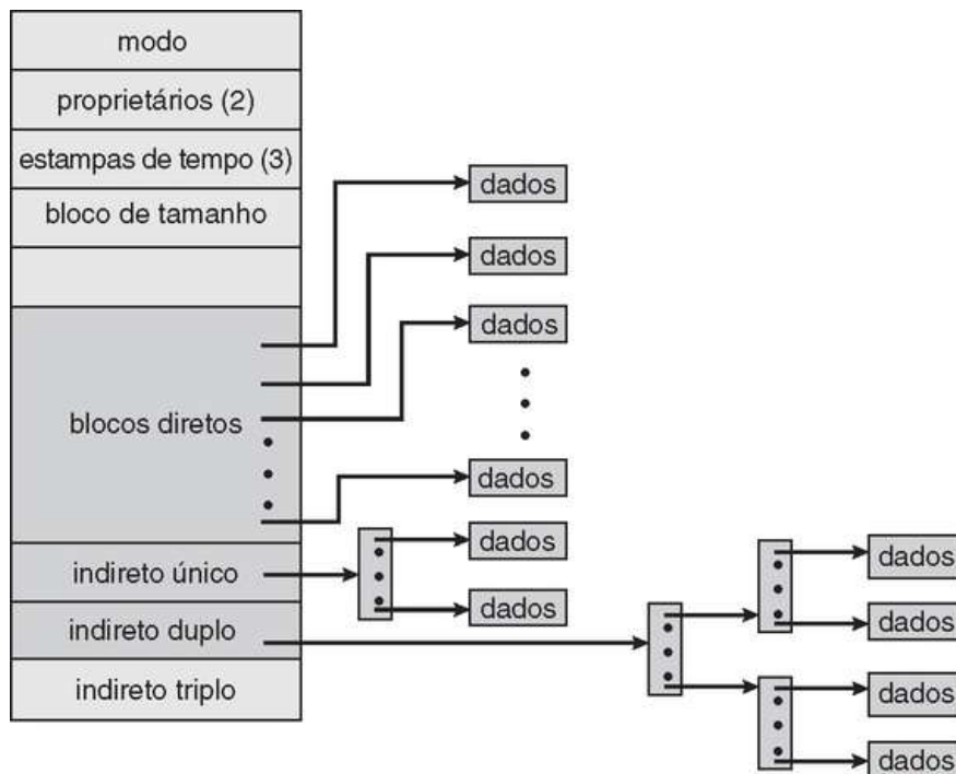
FIGURA 11.9 O inode do UNIX.
