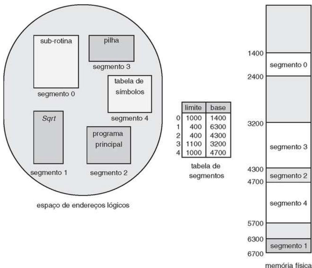
FIGURA 8.20 Exemplo de segmentação.
