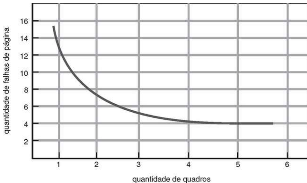
FIGURA 9.11 Gráfico para falhas de página versus quantidade de quadros.
