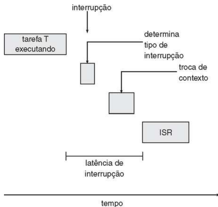
FIGURA 19.4 Latência de interrupção.
