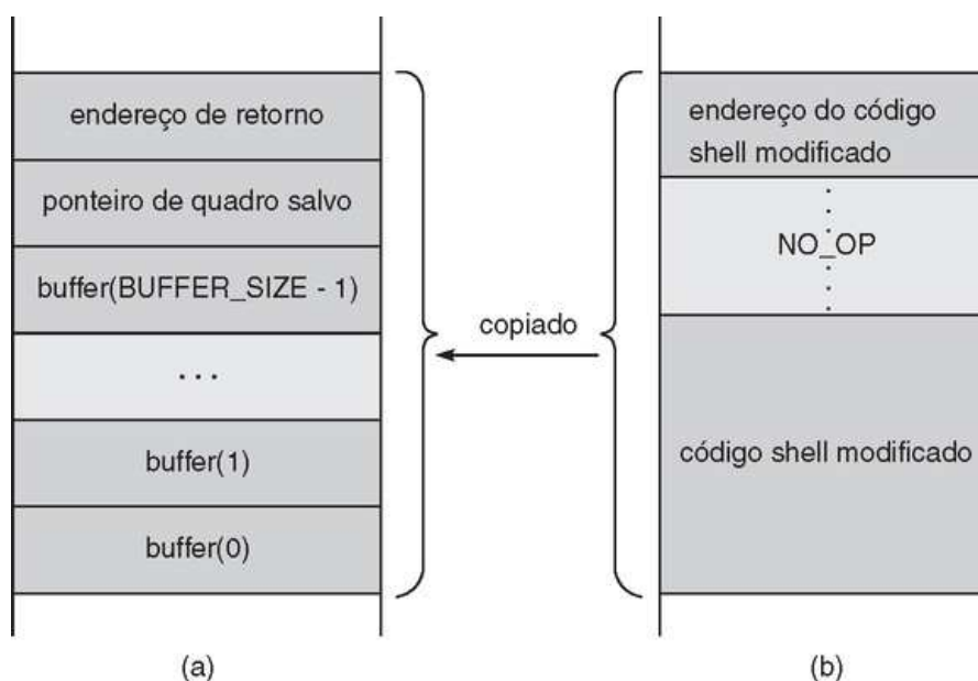
FIGURA 15.4 Quadro de pilha hipotético para a Figura 15.2 , antes (a) e depois (b).
