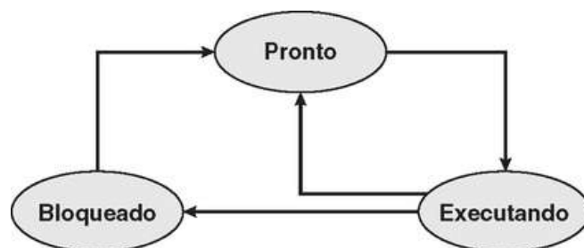
FIGURA 9.30 Diagrama de estado de thread para o Exercício 9.15 .
