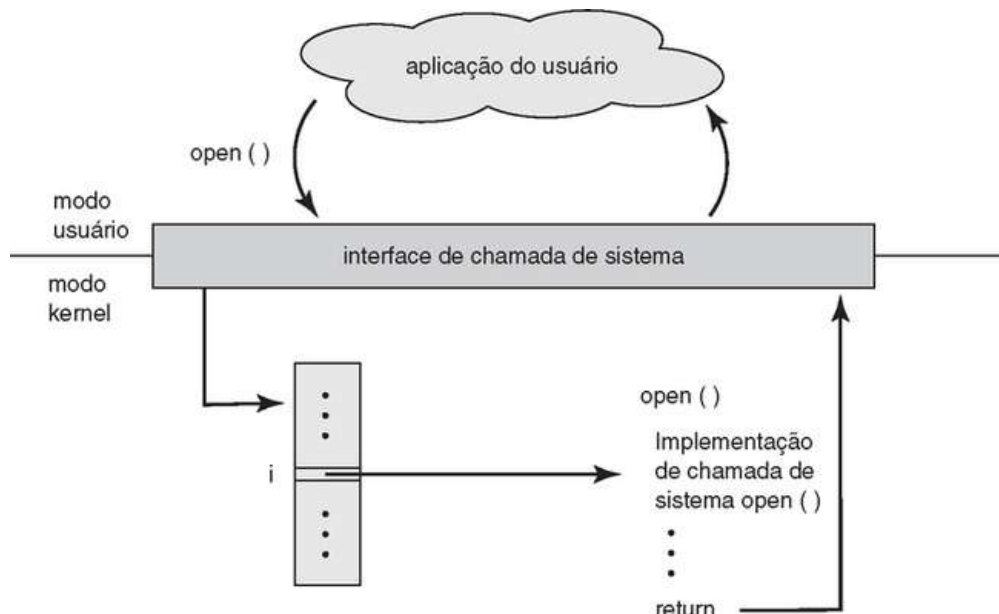
FIGURA 2.6 O tratamento de uma aplicação do usuário invocando a chamada de sistema open() .
