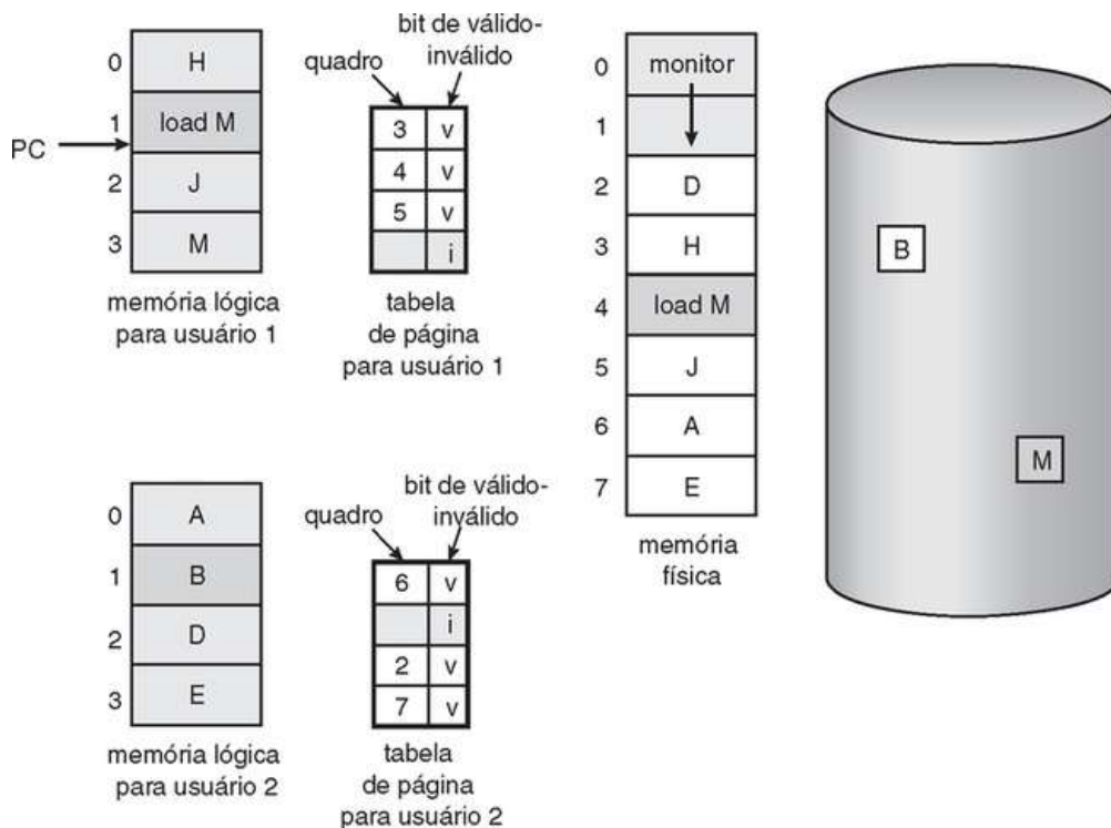
FIGURA 9.9 Necessidade de substituição de página.
