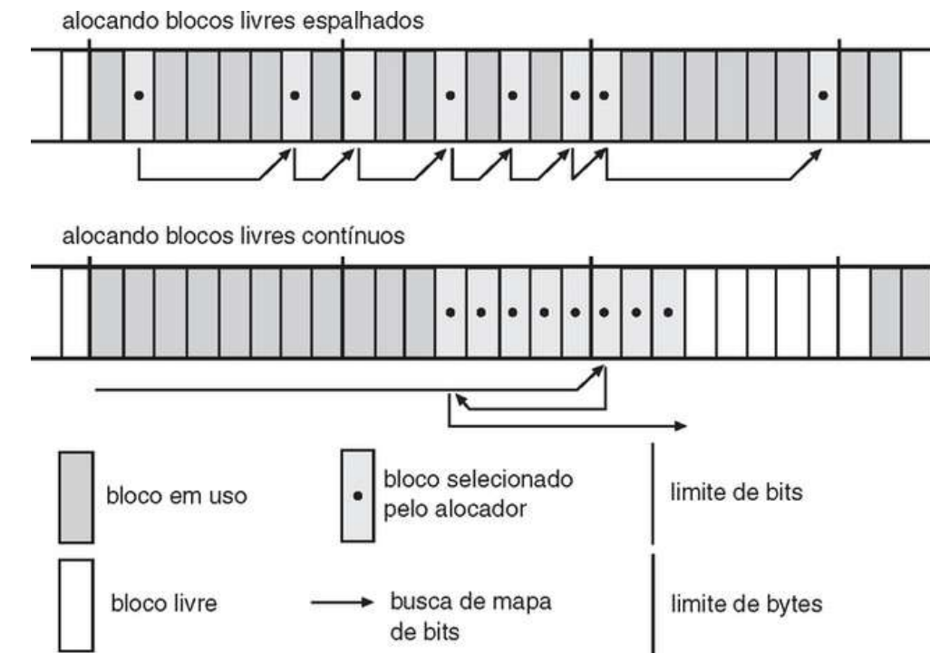
FIGURA 21.9 Políticas de alocação de bloco do ext2fs.
