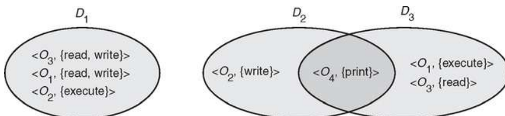
FIGURA 14.1 Sistema com três domínios de proteção.
