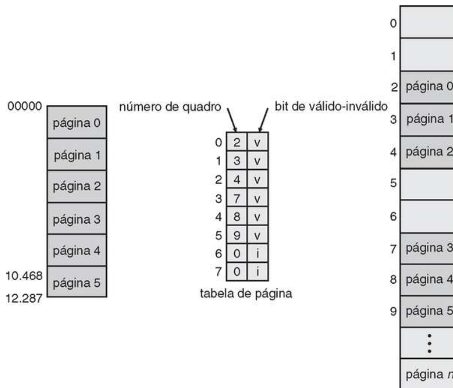
FIGURA 8.12 Bit válido (v) ou ínválido (i) em uma tabela de página.
