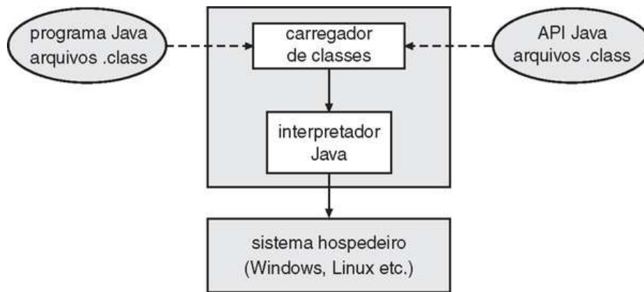
FIGURA 2.20 A máquina virtual Java (JVM).
