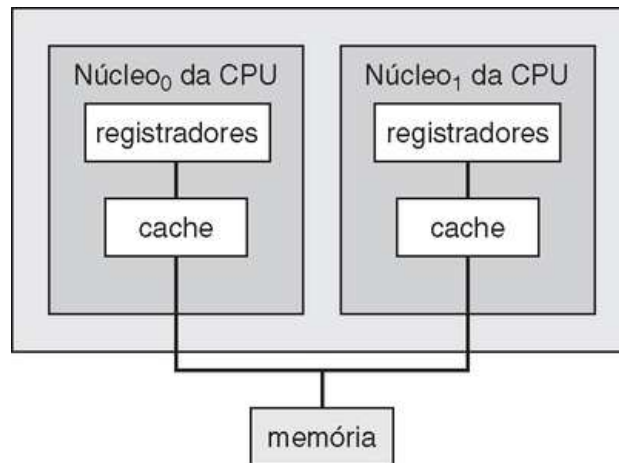
FIGURA 1.7 Um projeto dual-core com dois núcleos colocados no mesmo chip.
