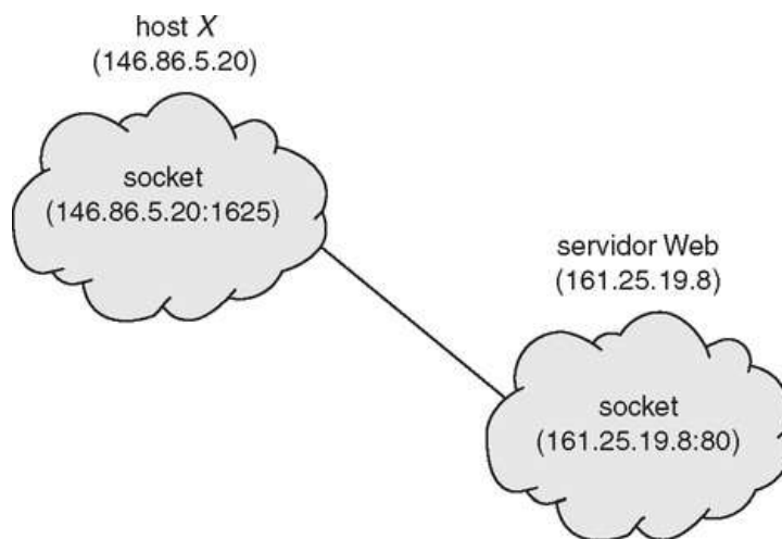
FIGURA 3.25 Comunicação usando sockets.
