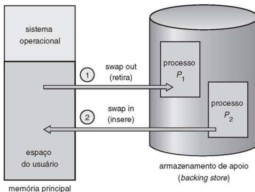
FIGURA 8.5 Swap de dois processos usando um disco como armazenamento de apoio.
