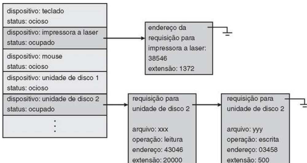
FIGURA 13.9 Tabela de status de dispositivo.
