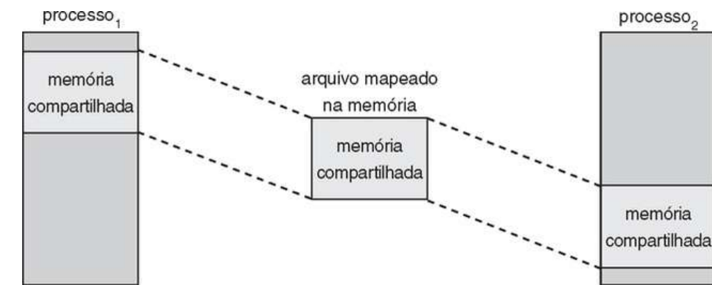
FIGURA 9.24 Memória compartilhada no Windows usando E/S mapeada na memória.
