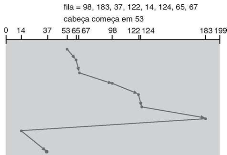
FIGURA 12.8 Escalonamento de disco C-LOOK.
