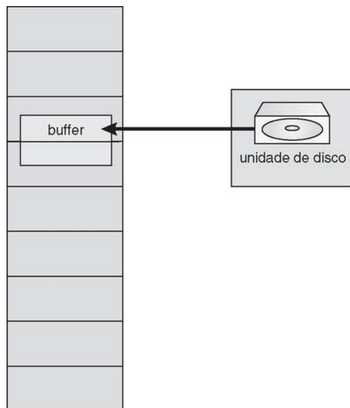
FIGURA 9.28 O motivo pelo qual os quadros usados para E/S precisam estar na memória.
