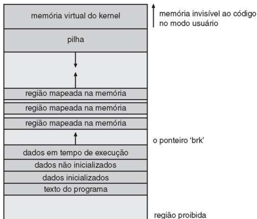
FIGURA 21.8 Layout da memória para os programas ELF.
