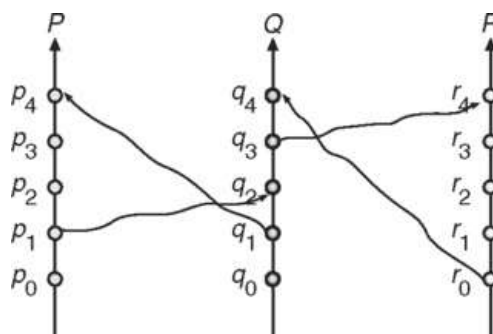
FIGURA 18.1 Tempo relativo para três processos simultâneos.
