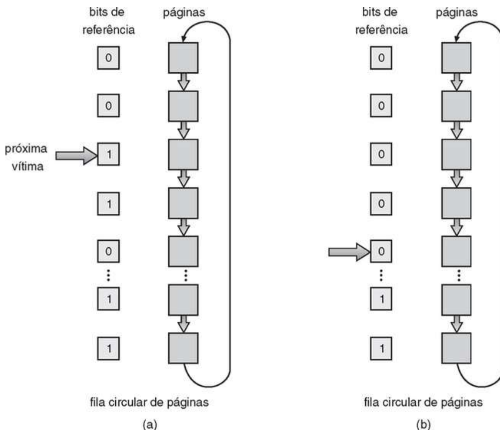
FIGURA 9.17 Algoritmo de substituição de página pela segunda chance (relógio).
