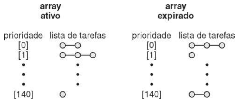
FIGURA 5.16 Lista de tarefas indexadas de acordo com a prioridade.
