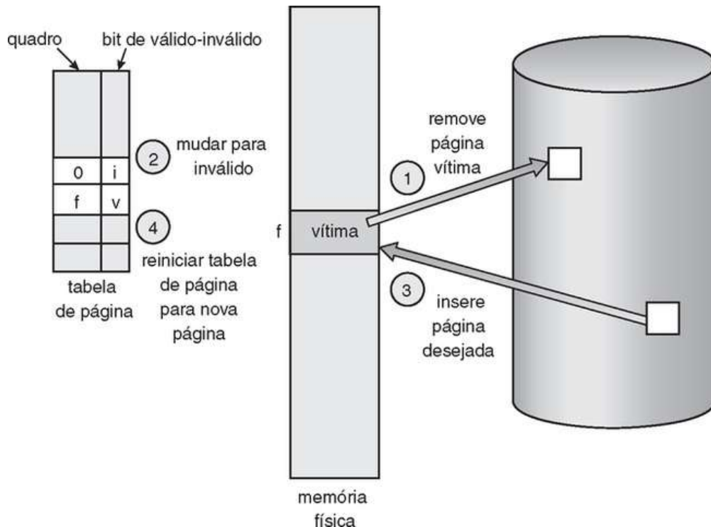
FIGURA 9.10 Substituição de página.
