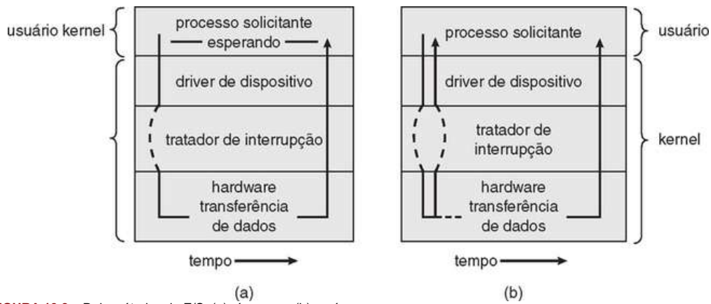
FIGURA 13.8 Dois métodos de E/S: (a) síncrona e (b) assíncrona.
