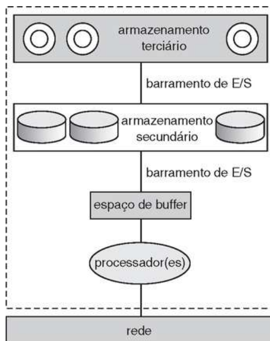
FIGURA 20.1 Recursos em um servidor de arquivos.
