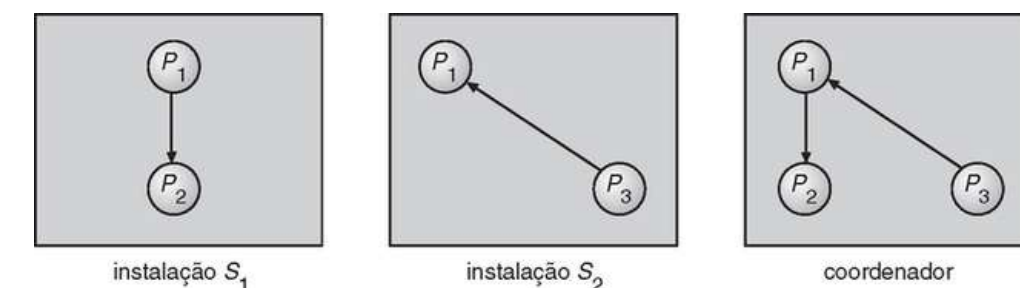
FIGURA 18.5 Grafos de espera local e global.
