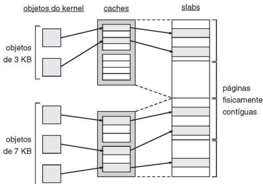
FIGURA 21.7 Alocador de slabs no Linux.
