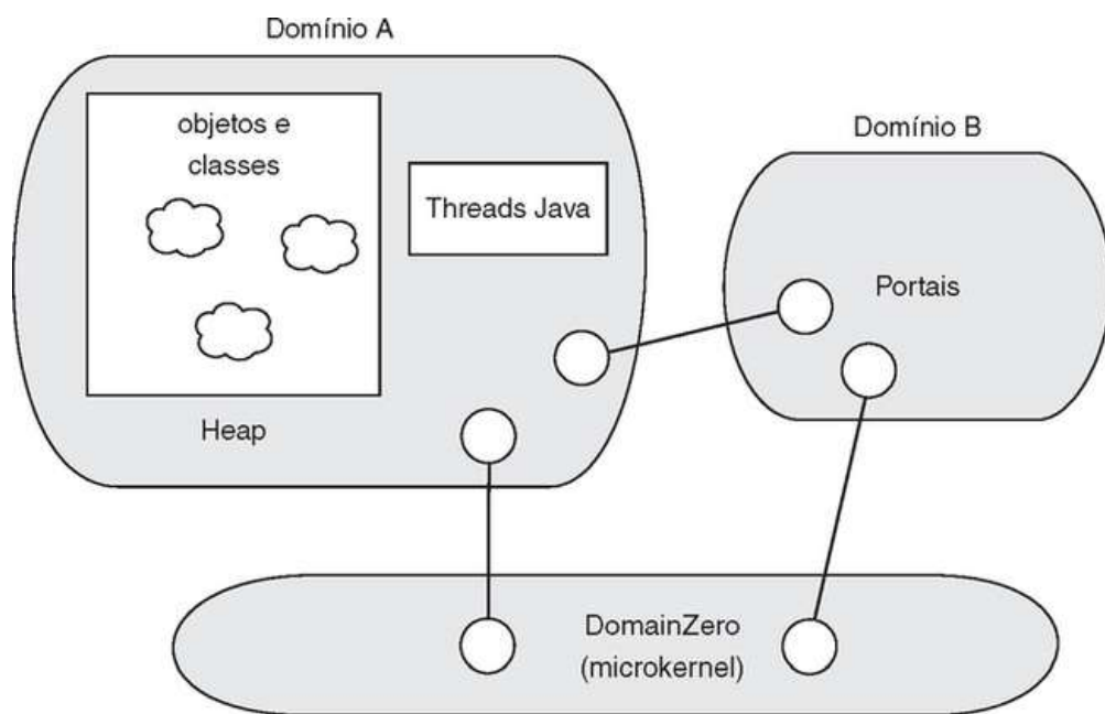
FIGURA 2.22 O sistema operacional JX.
