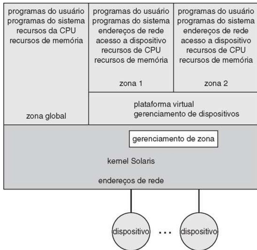
FIGURA 2.19 Solaris 10 com dois contêineres.
